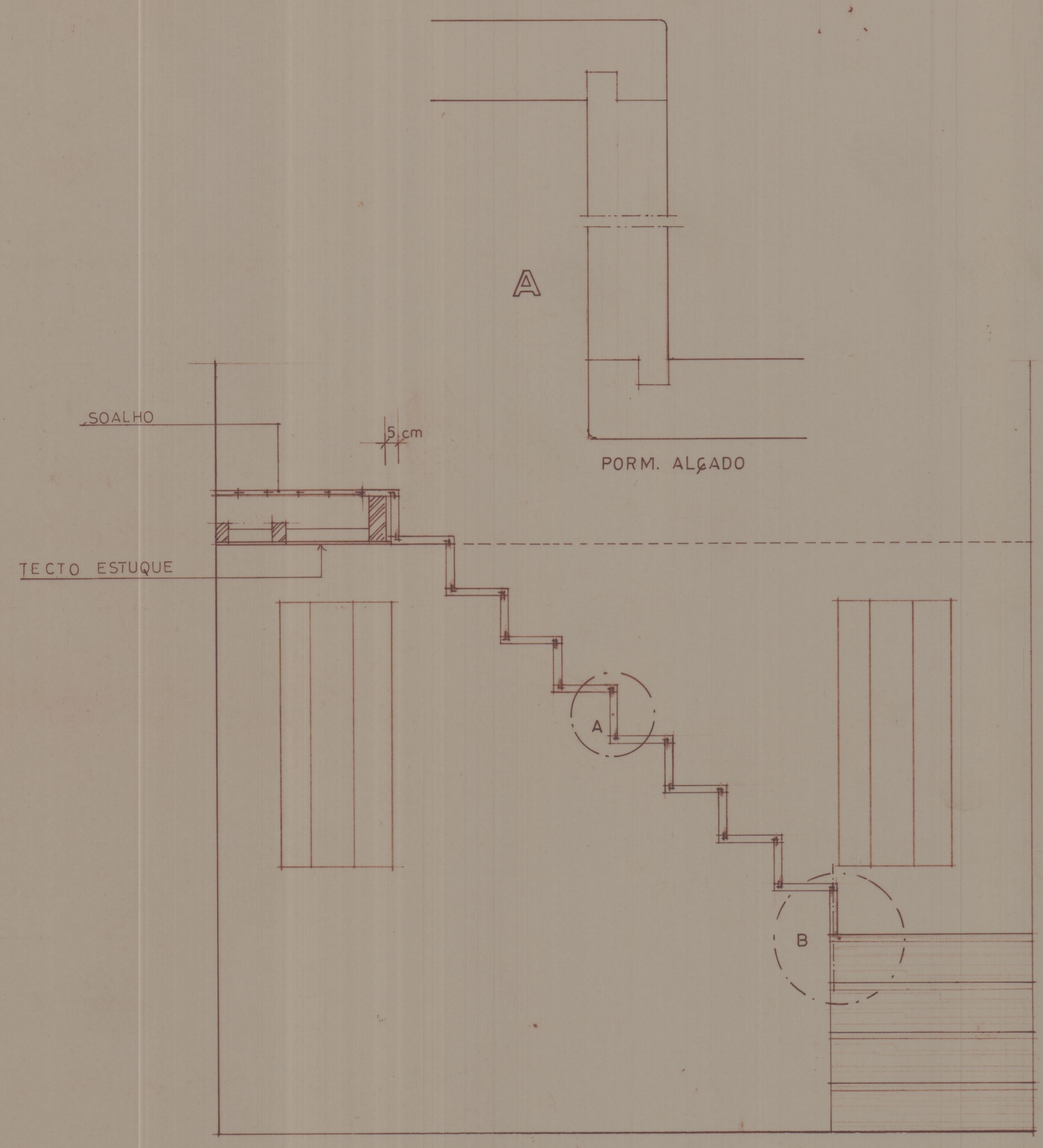
ALÇADO
