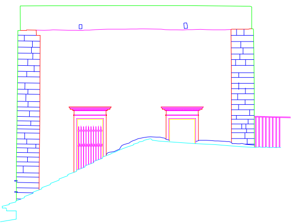
ALÇADOS NORTE
