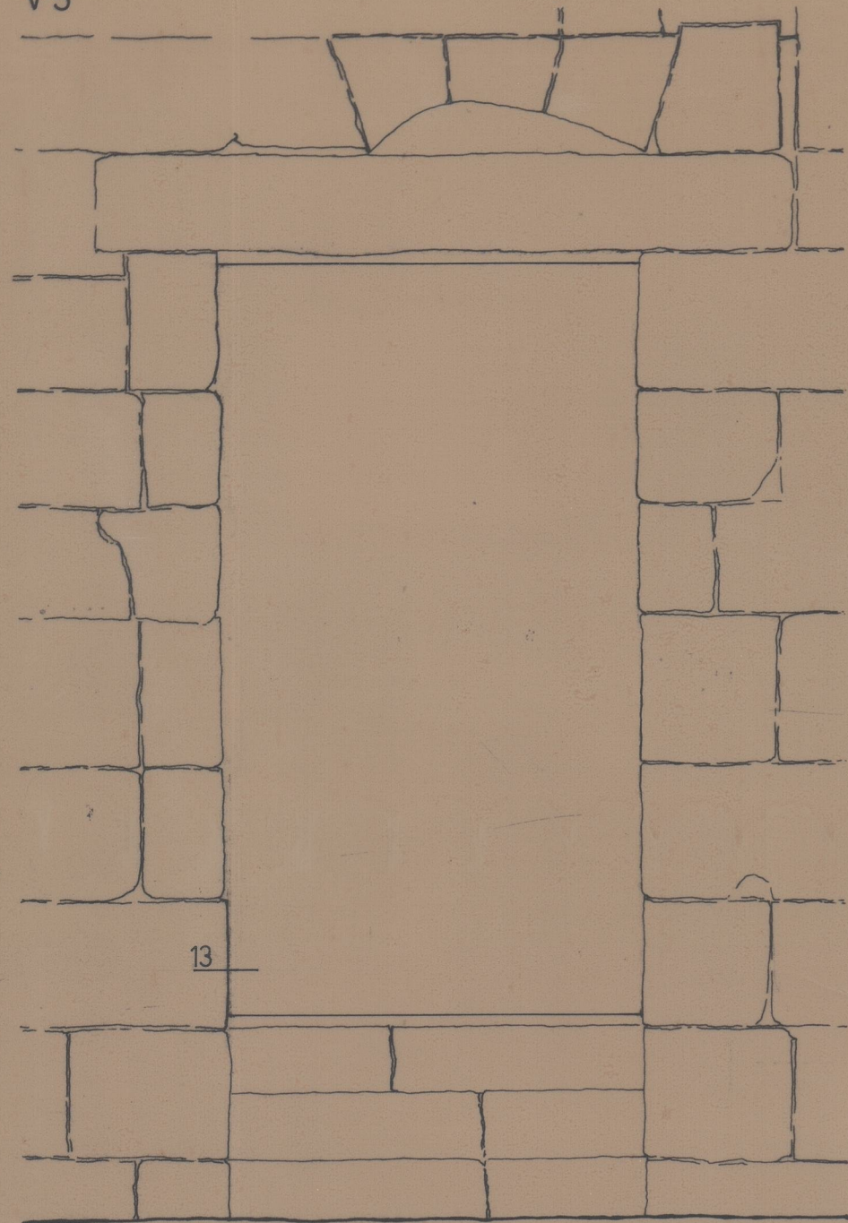
PF1 ALÇADO EXT.
