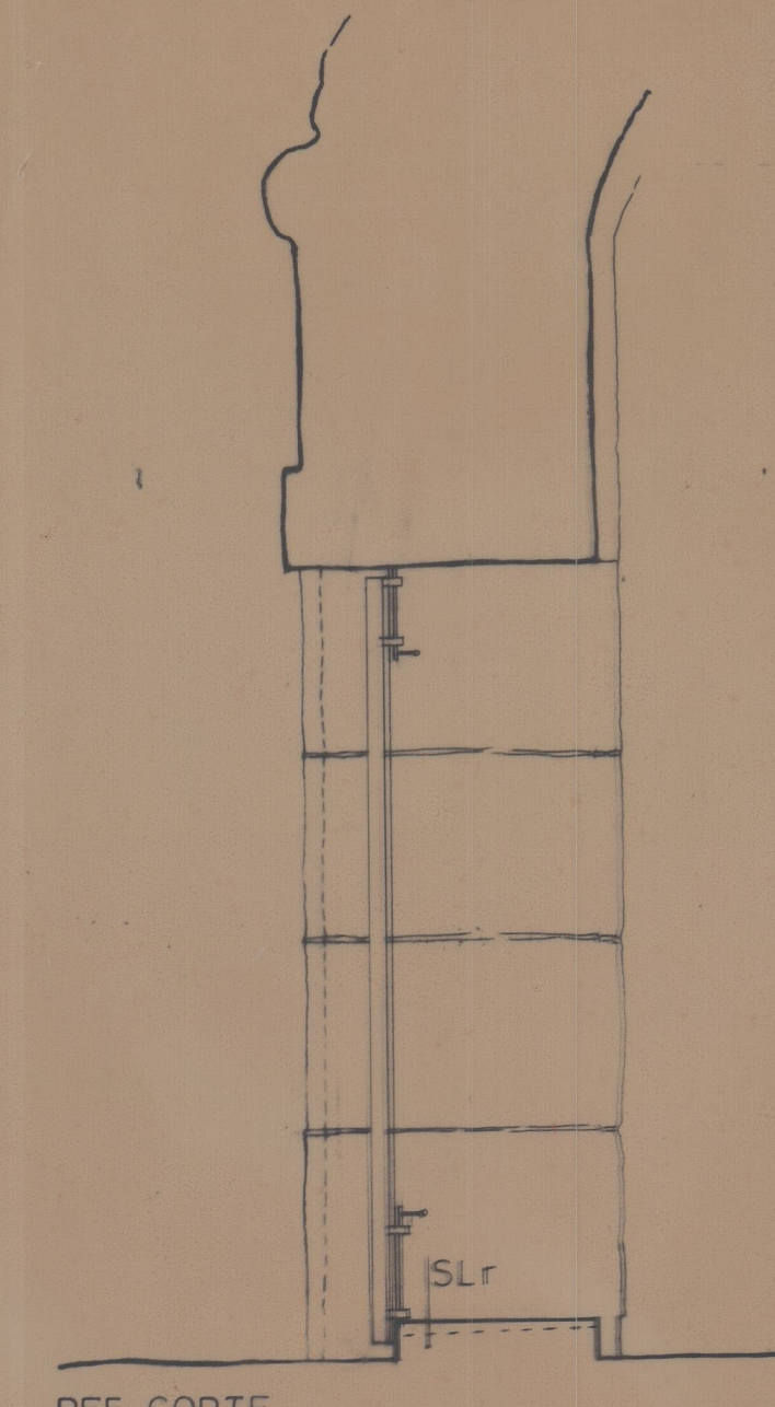
PF5 CORTE
