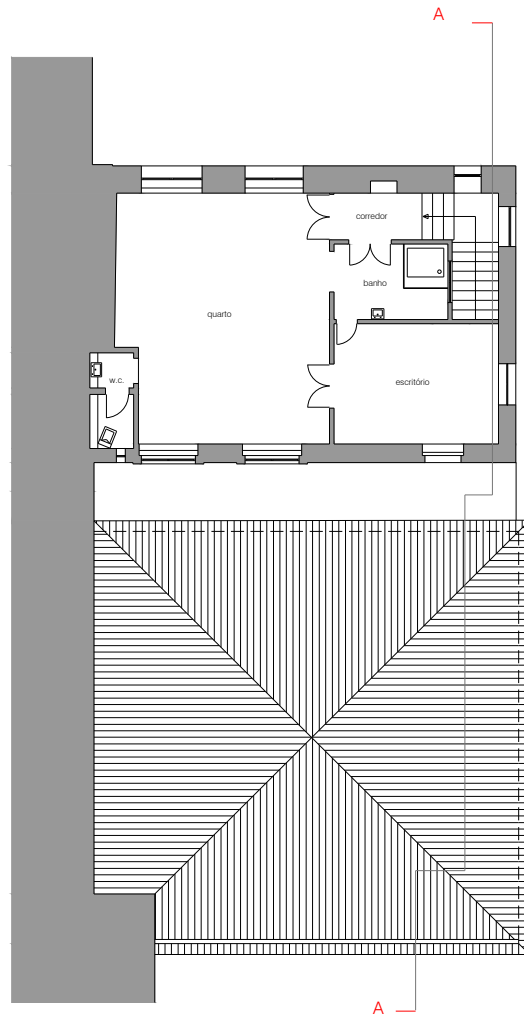
Planta do Piso 2 e Cobertura
