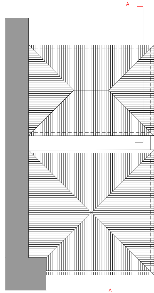
Planta das Coberturas
