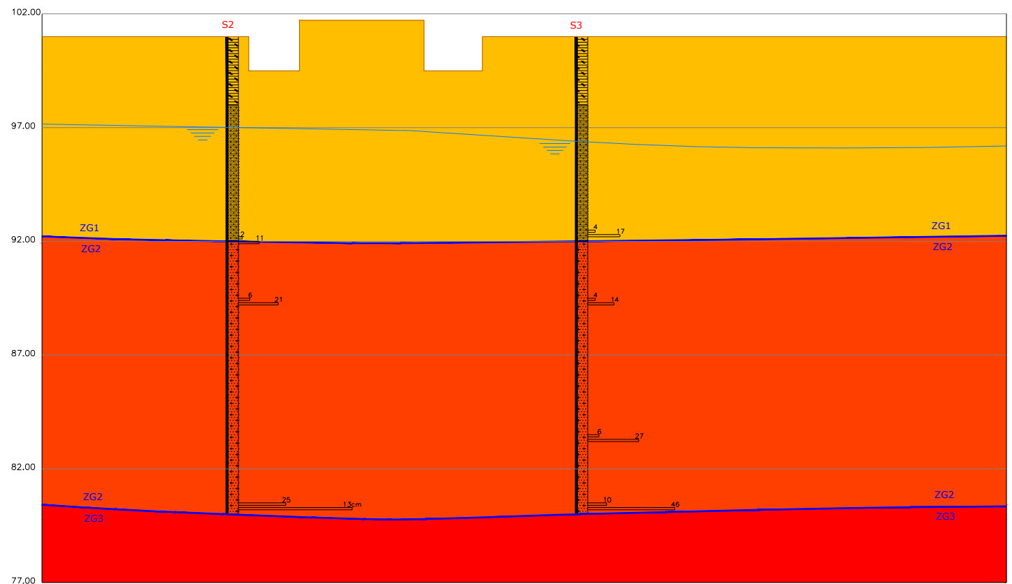
PERFIL INTERPRETATIVO A-B
