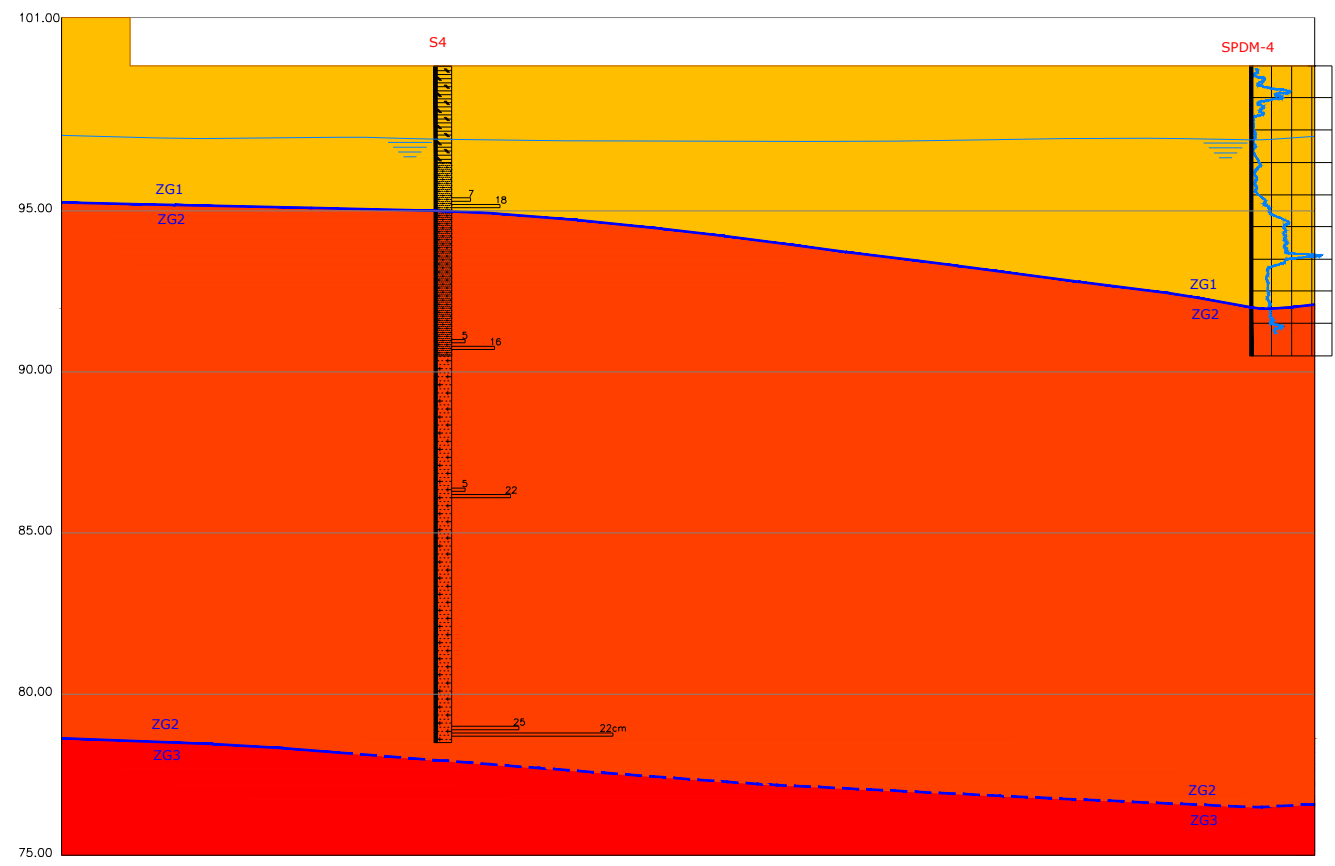
PERFIL INTERPRETATIVO G-F
