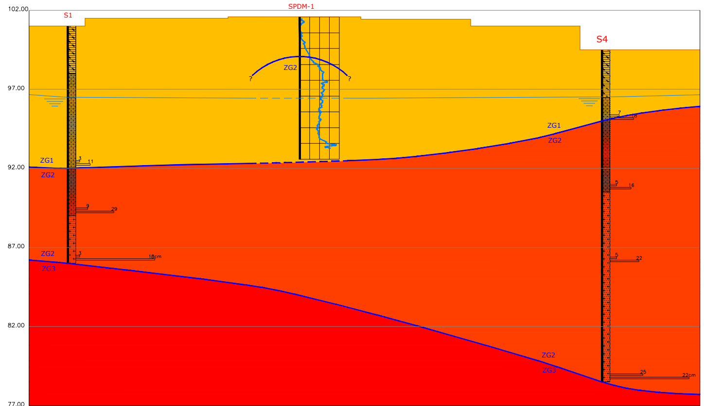
PERFIL INTERPRETATIVO C-D
