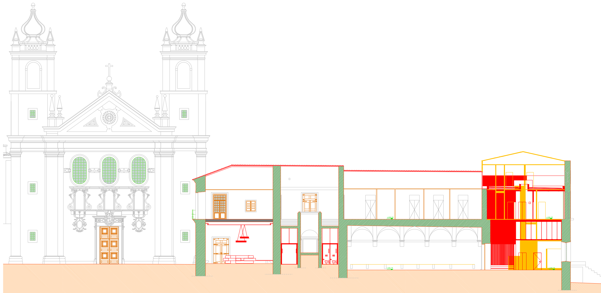
Corte CC
