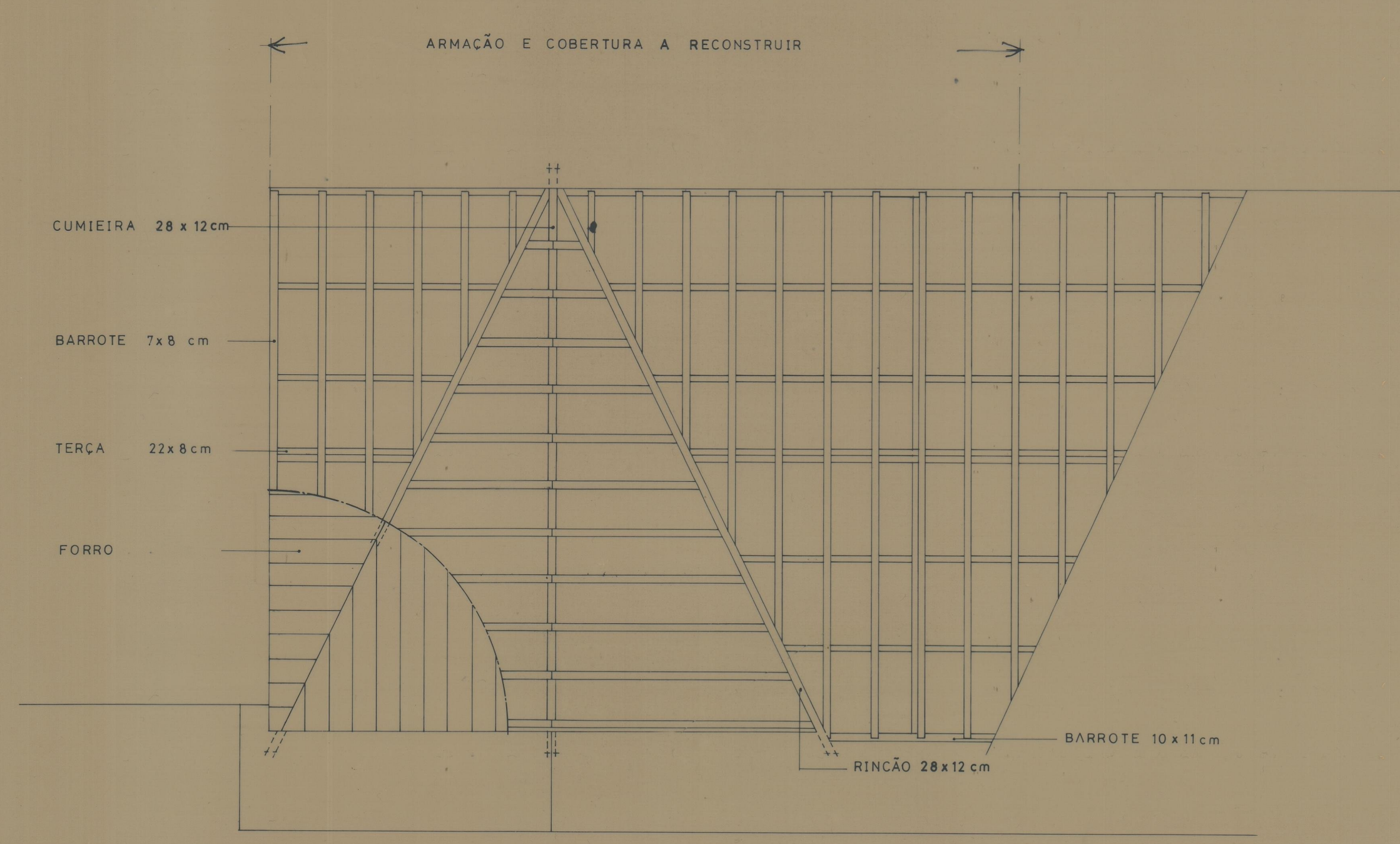
PORM. K PLANTA
