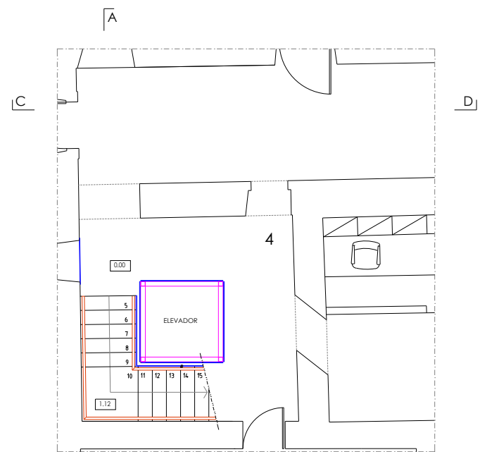
B PLANTA DO PISO 0
