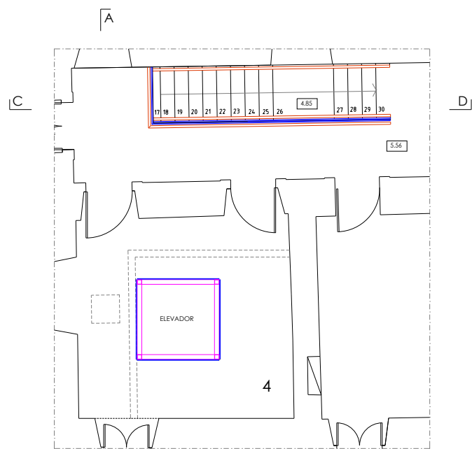
B PLANTA DO PISO 2
