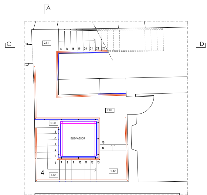
B PLANTA DO PISO INTERMÉDIO
