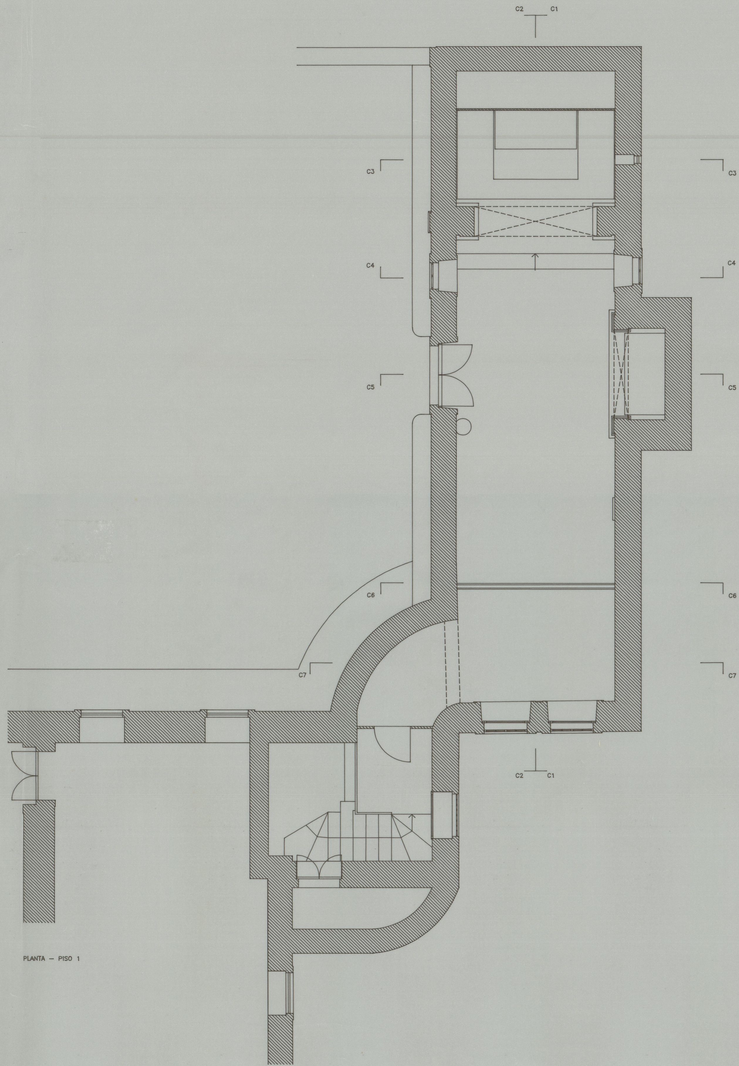
PLANTA - PISO 0
