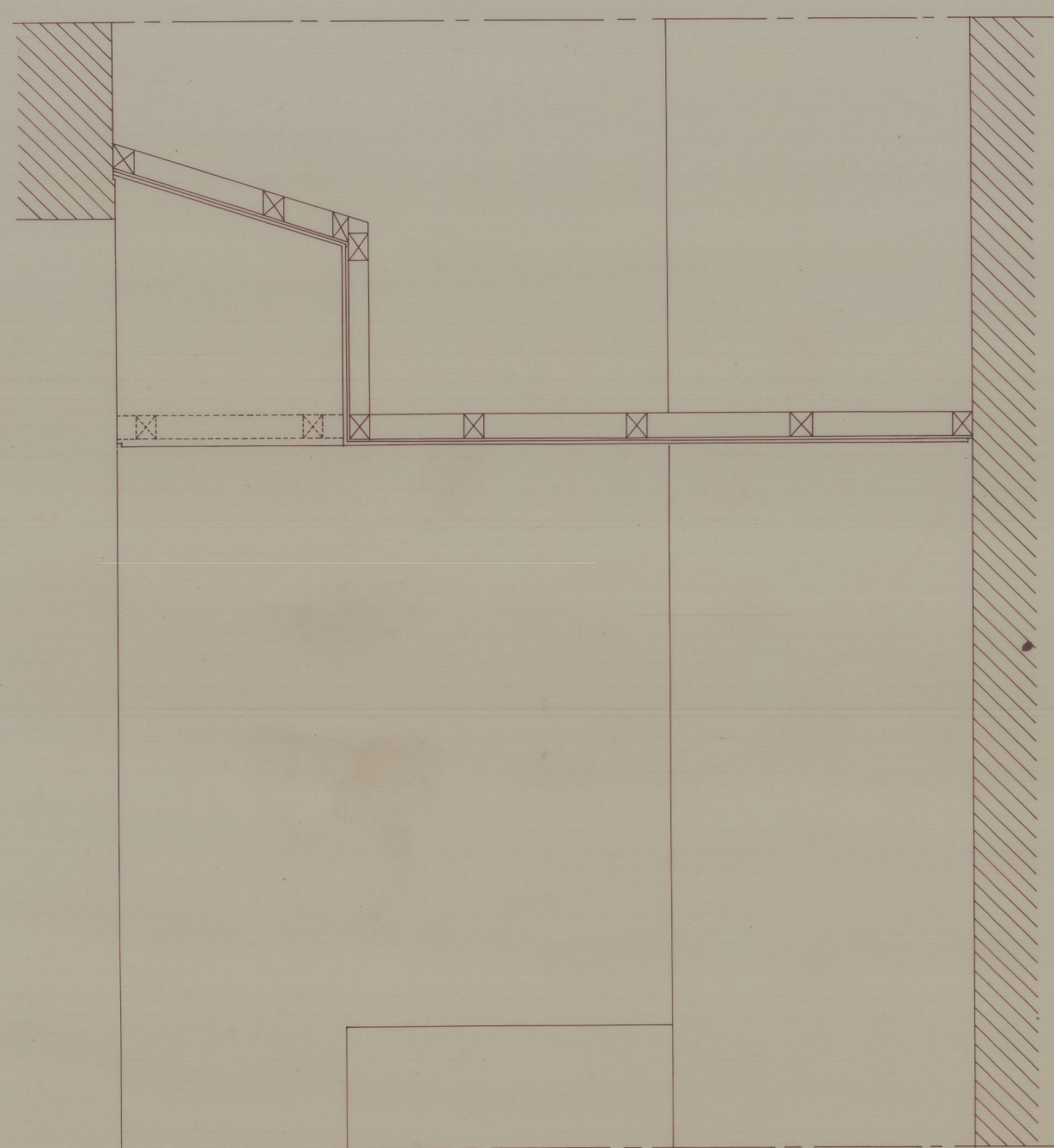
CORTE E.E
