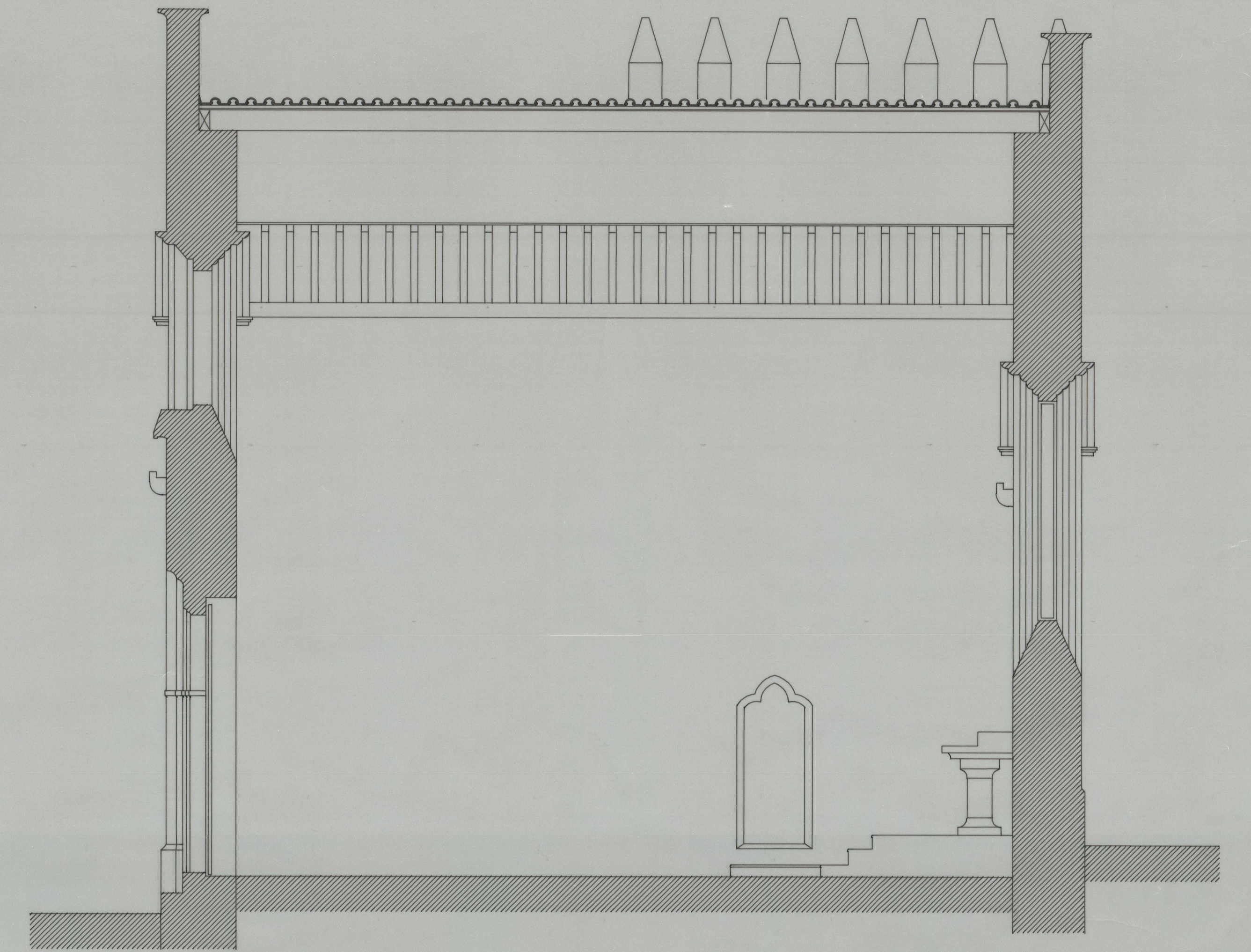
CORTE 2.2
