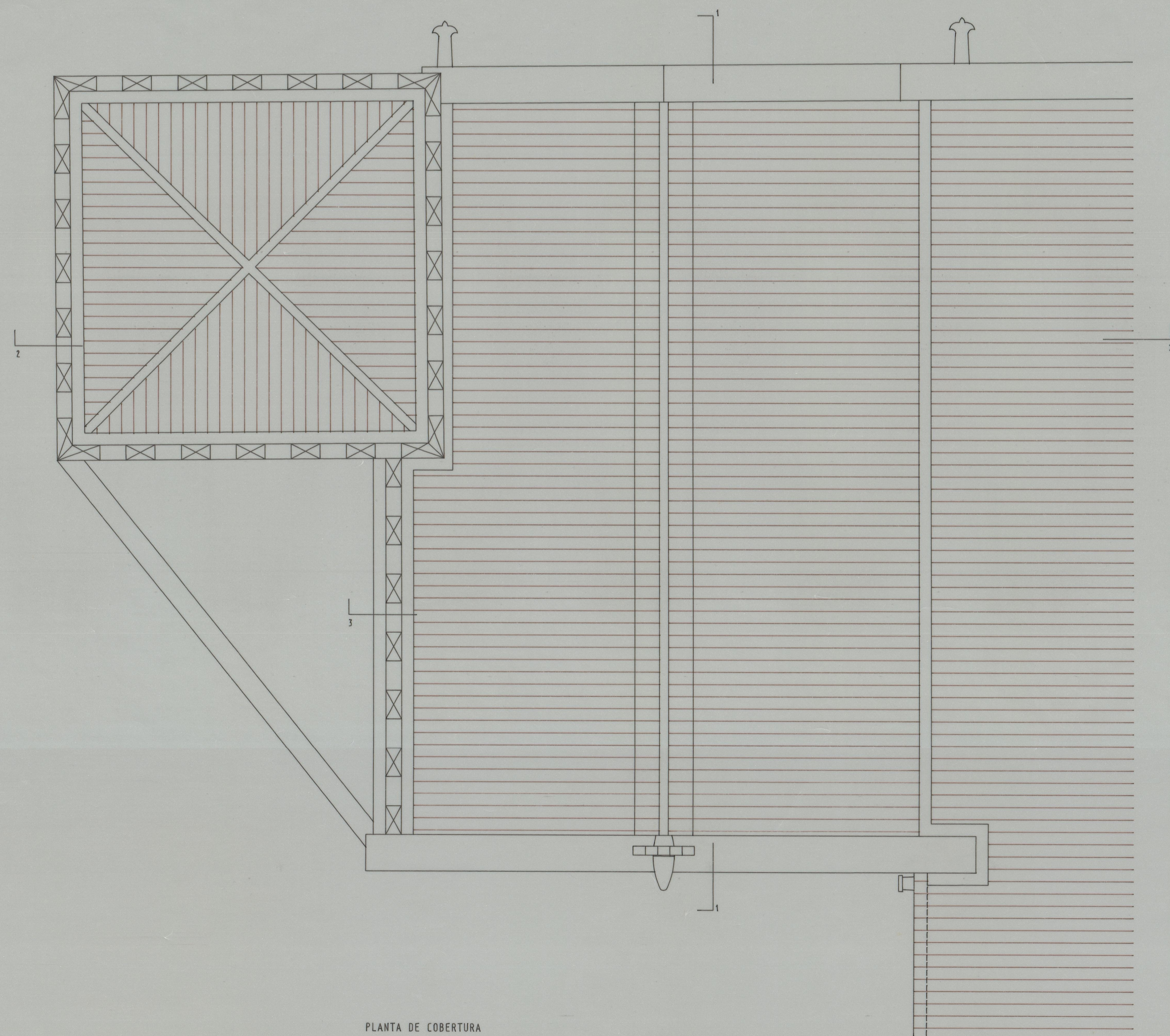
PLANTA DE COBERTURA
