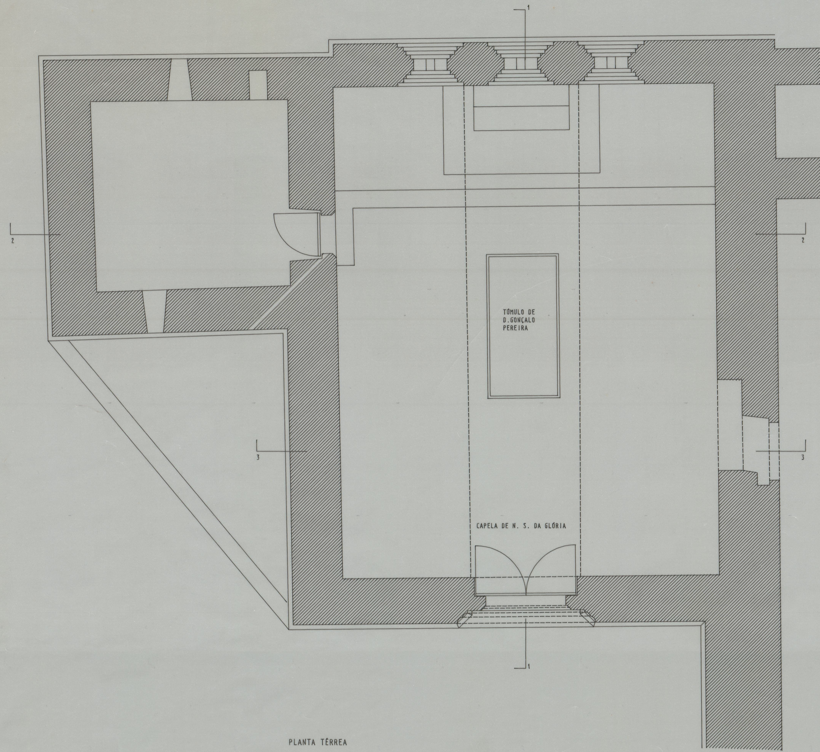
PLANTA TERREA
