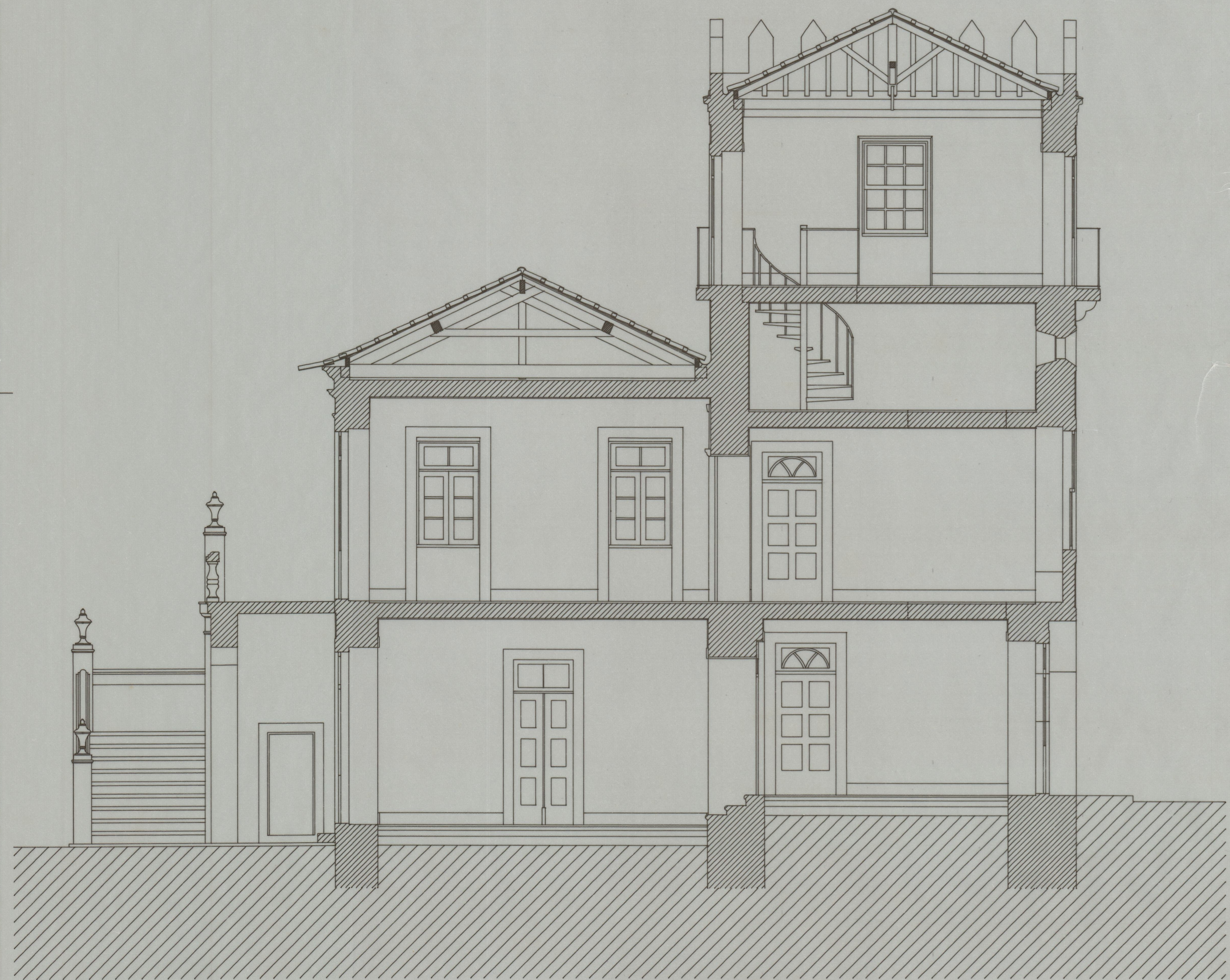
CORTE 3
