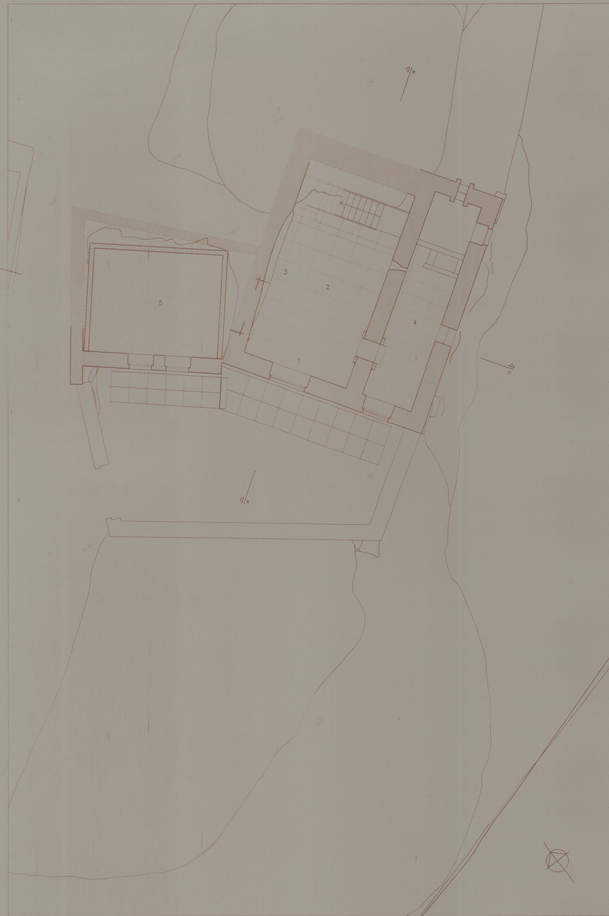
PLANTA PISO 1
