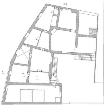
PLANTA DO 1º ANDAR
