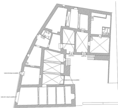
PLANTA DO RÉS - DO - CHÃO
