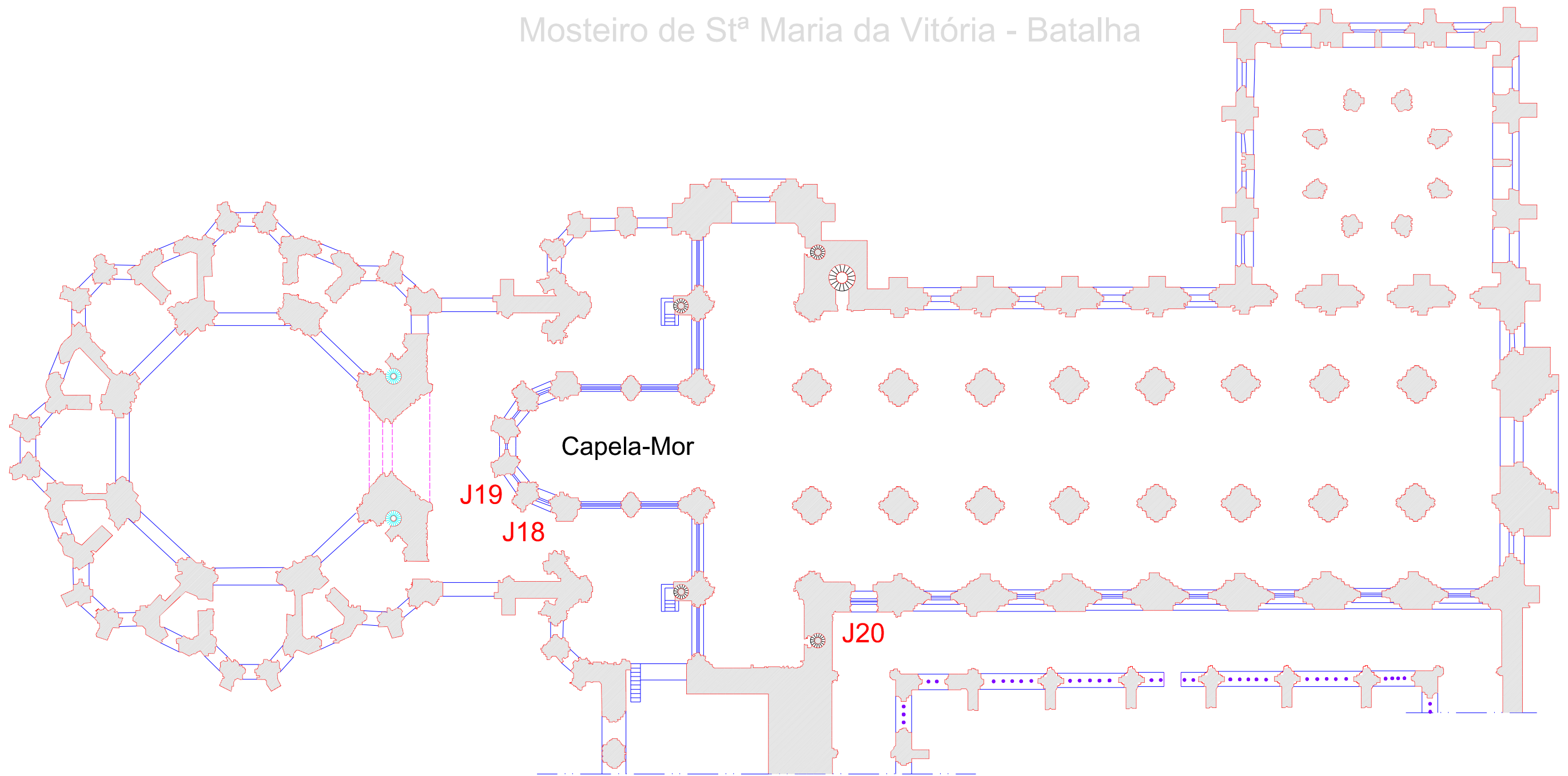
PLANTA DE IDENTIFICAÇÃO DOS PISOS INTERMÉDIO - VITRAIS
