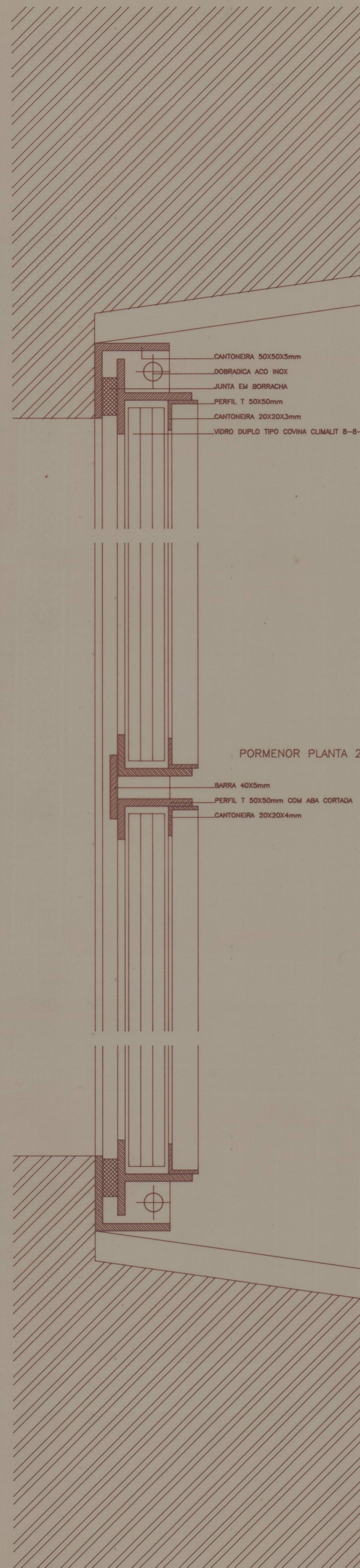
PORMENOR PLANTA 22
