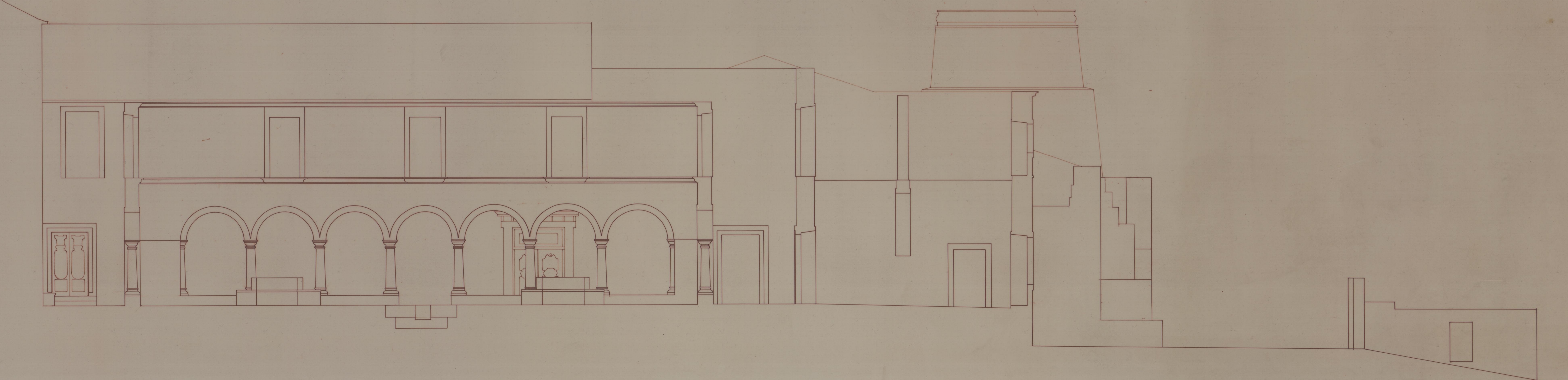
CORTE ALÇADO 4-4
