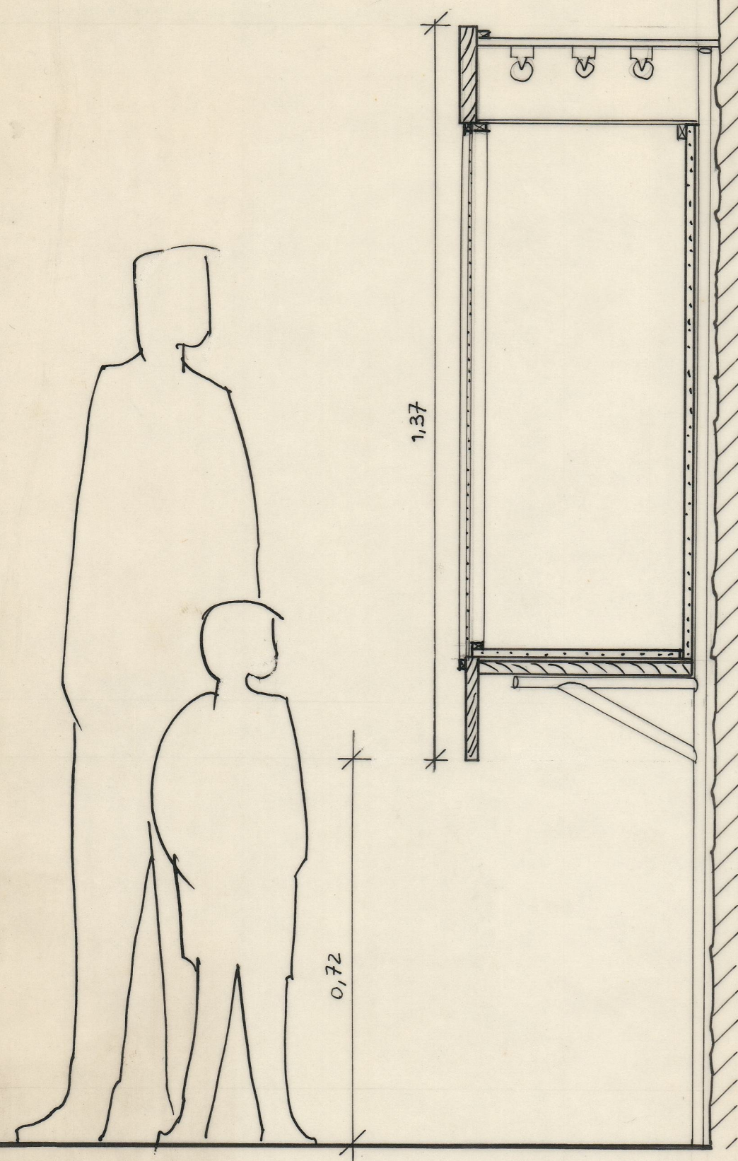
CORTE ESC 1/10
