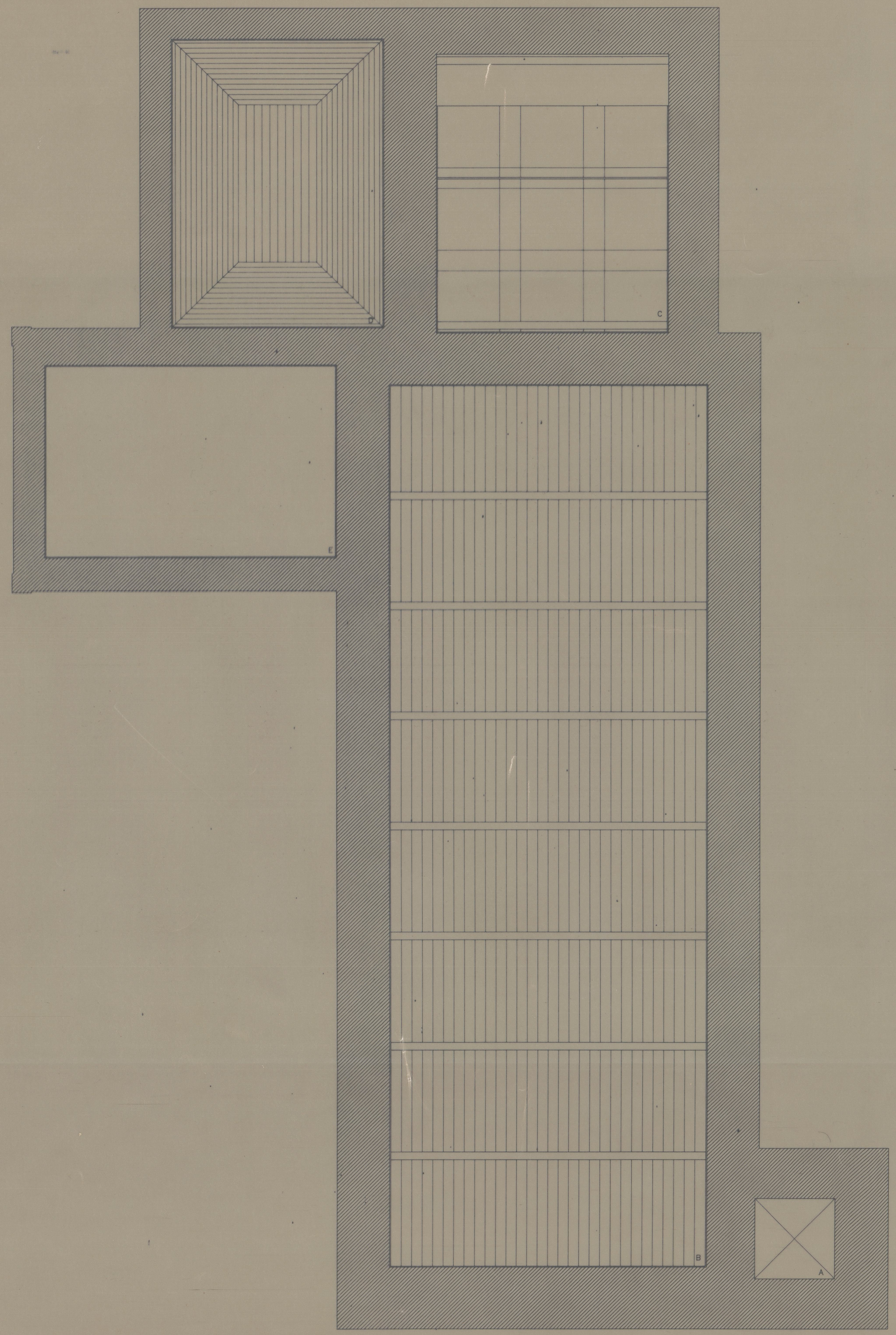
PLANTA DE TECTOS
