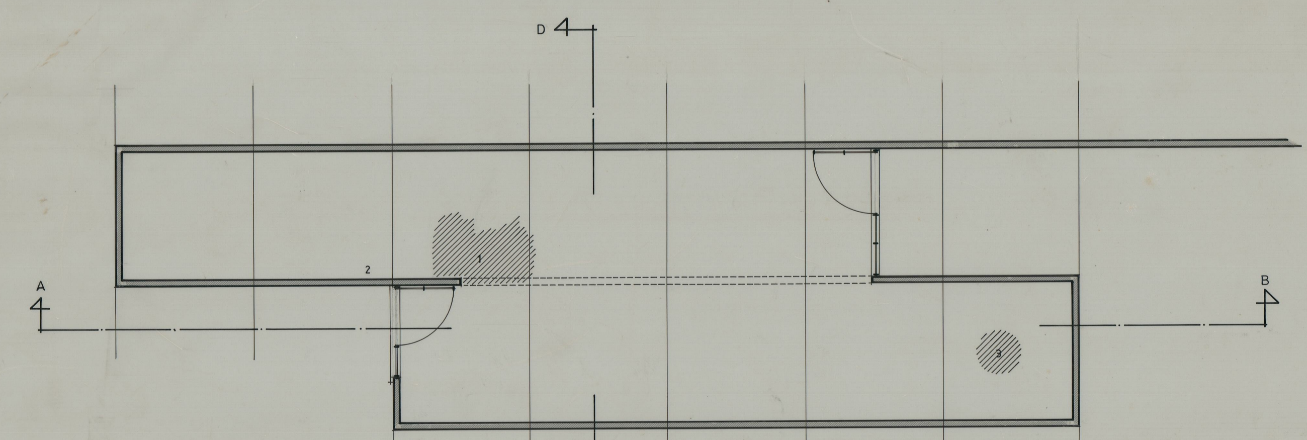
PLANTA
