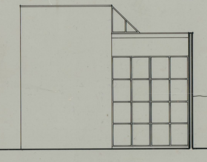
ALÇADO LAT. DIREITO
