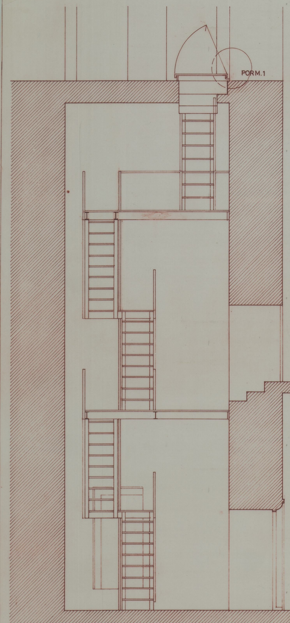
CORTE 22
