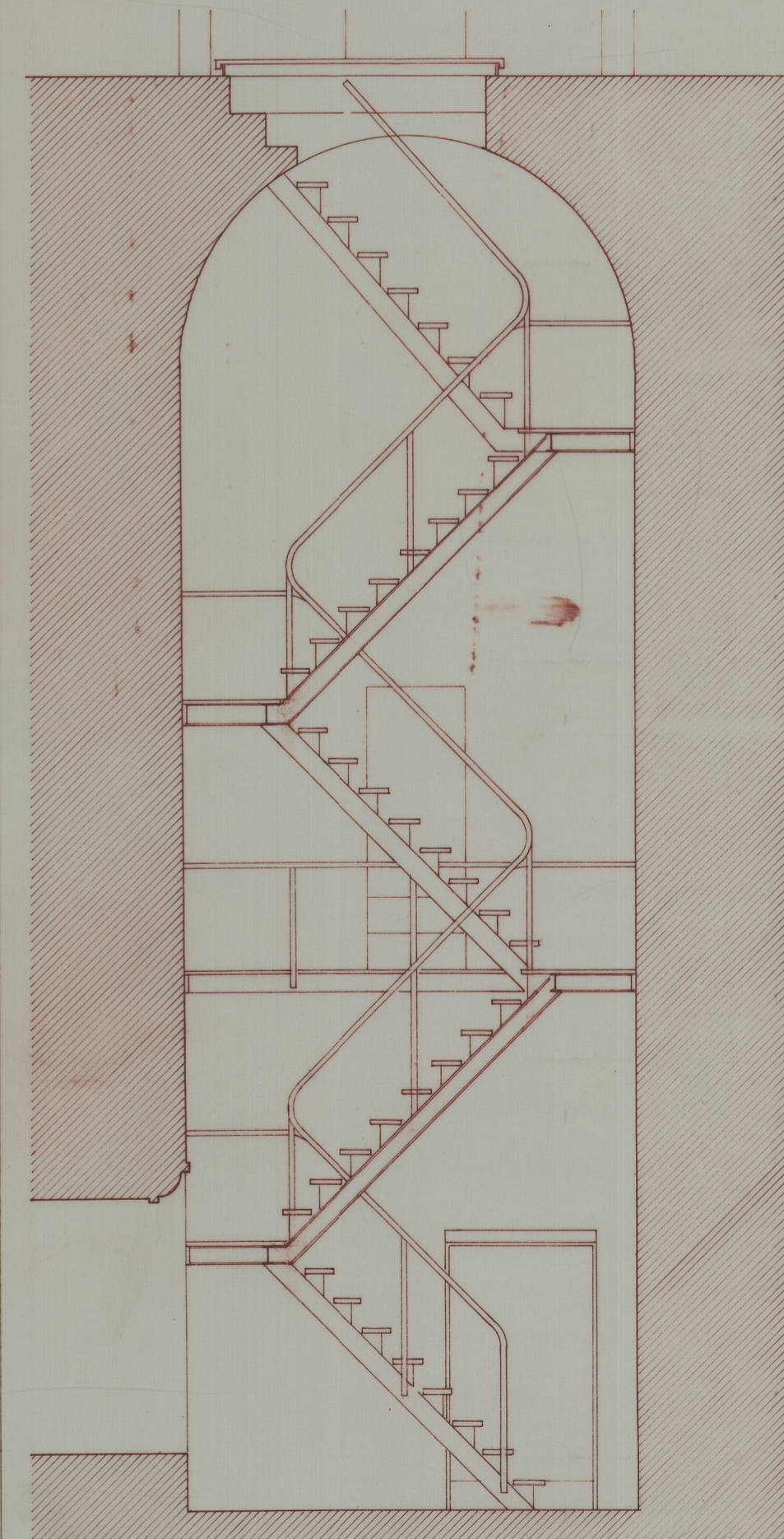
CORTE 22
