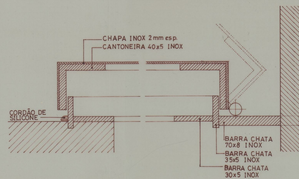
PORM.1 esc. 1:2
