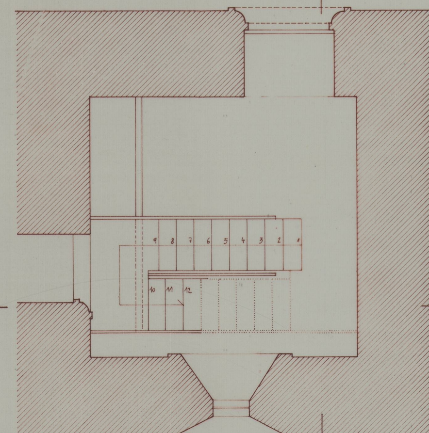
PLANTA cota 0,00
