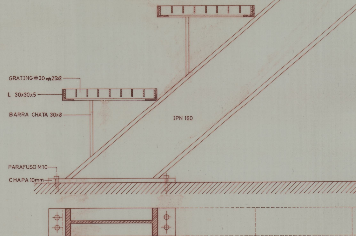
PORM. ESCADA METÁLICA esc. 1:2
