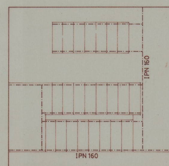
ESQUEMA ESTRUTURAL cota 8,64
