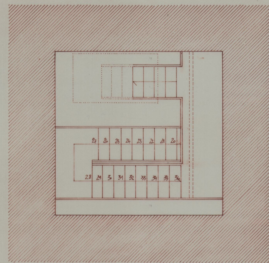
PLANTA cota 8,64
