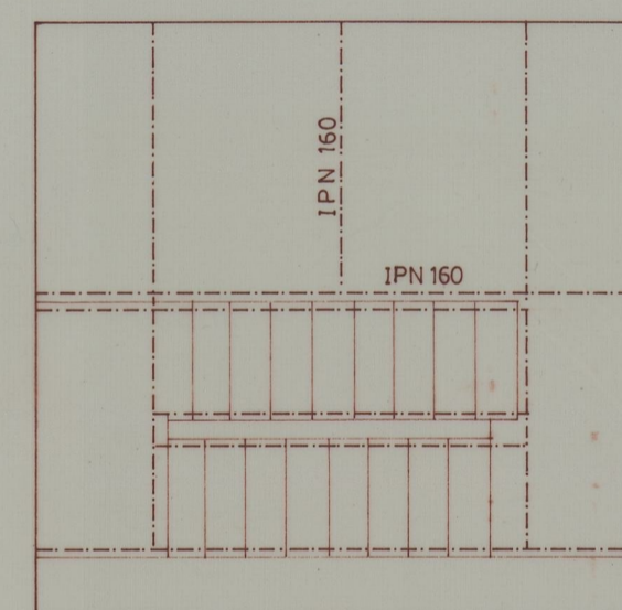
ESQUEMA ESTRUTURAL cota 4,32
