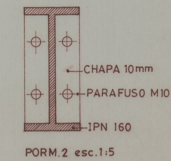
PORM.2 esc. 1:5
