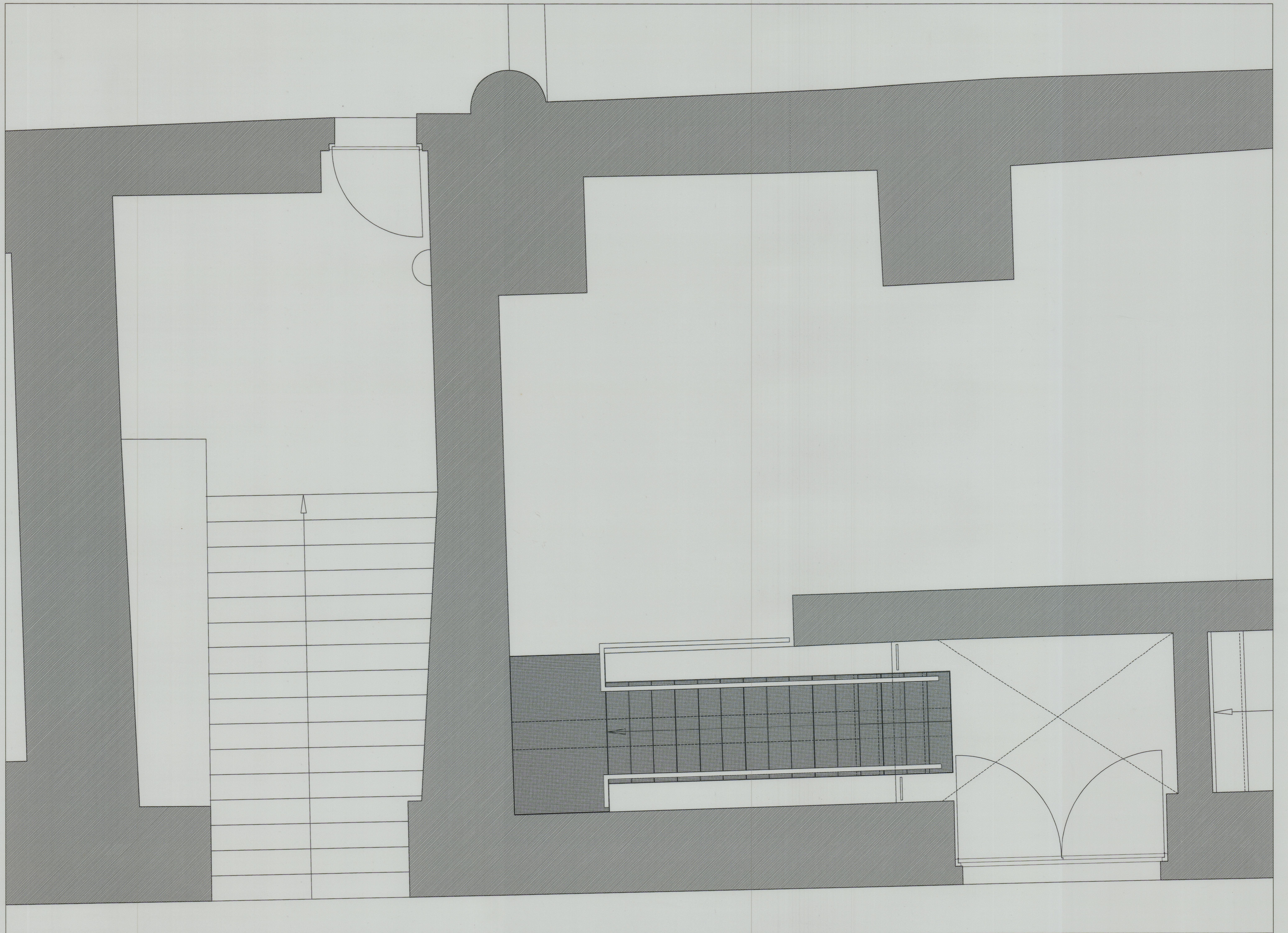
PLANTA DA ESCADA DE ACESSO AO CÔRO. PROPOSTO ESC:1/20
