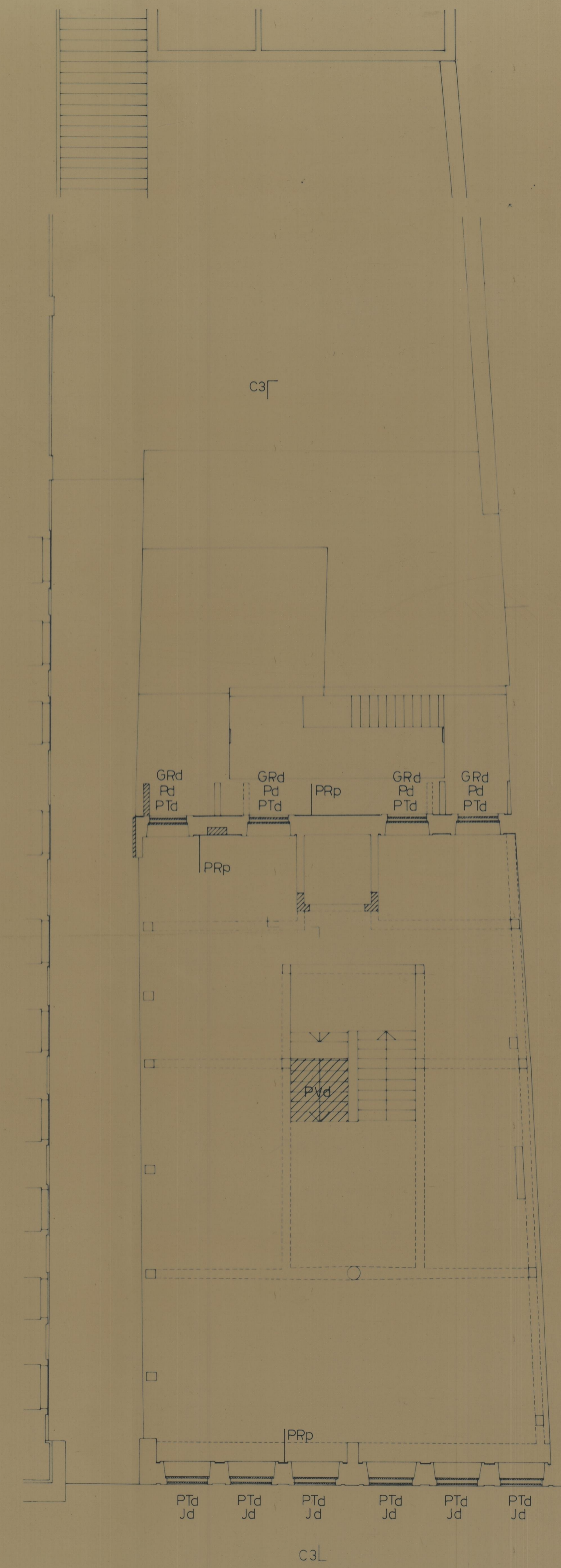
PLANTA PISO 3
