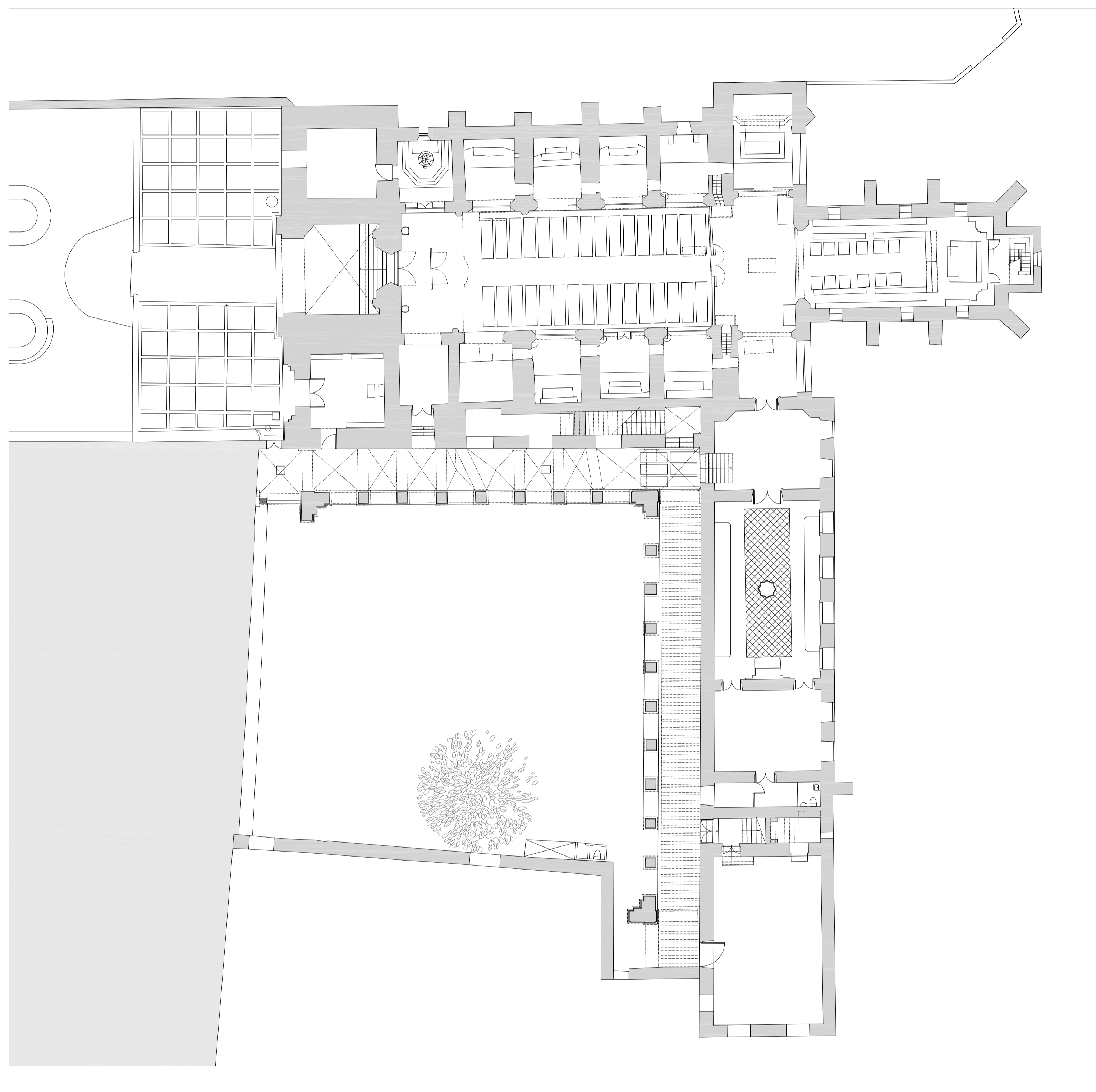
PLANTA DO PISO TÉRREO EXISTENTE
