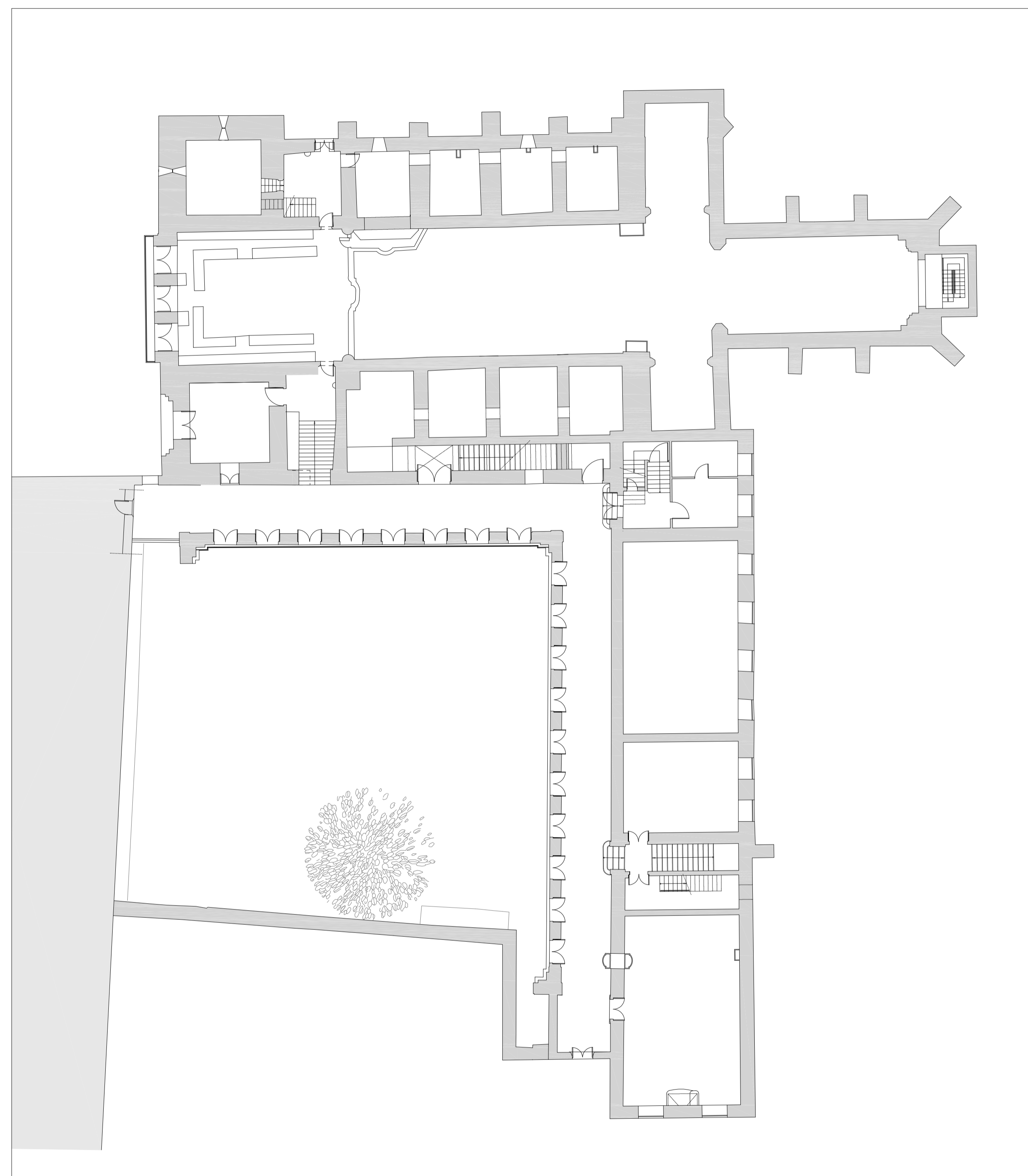
PLANTA DO 1º ANDAR EXISTENTE
