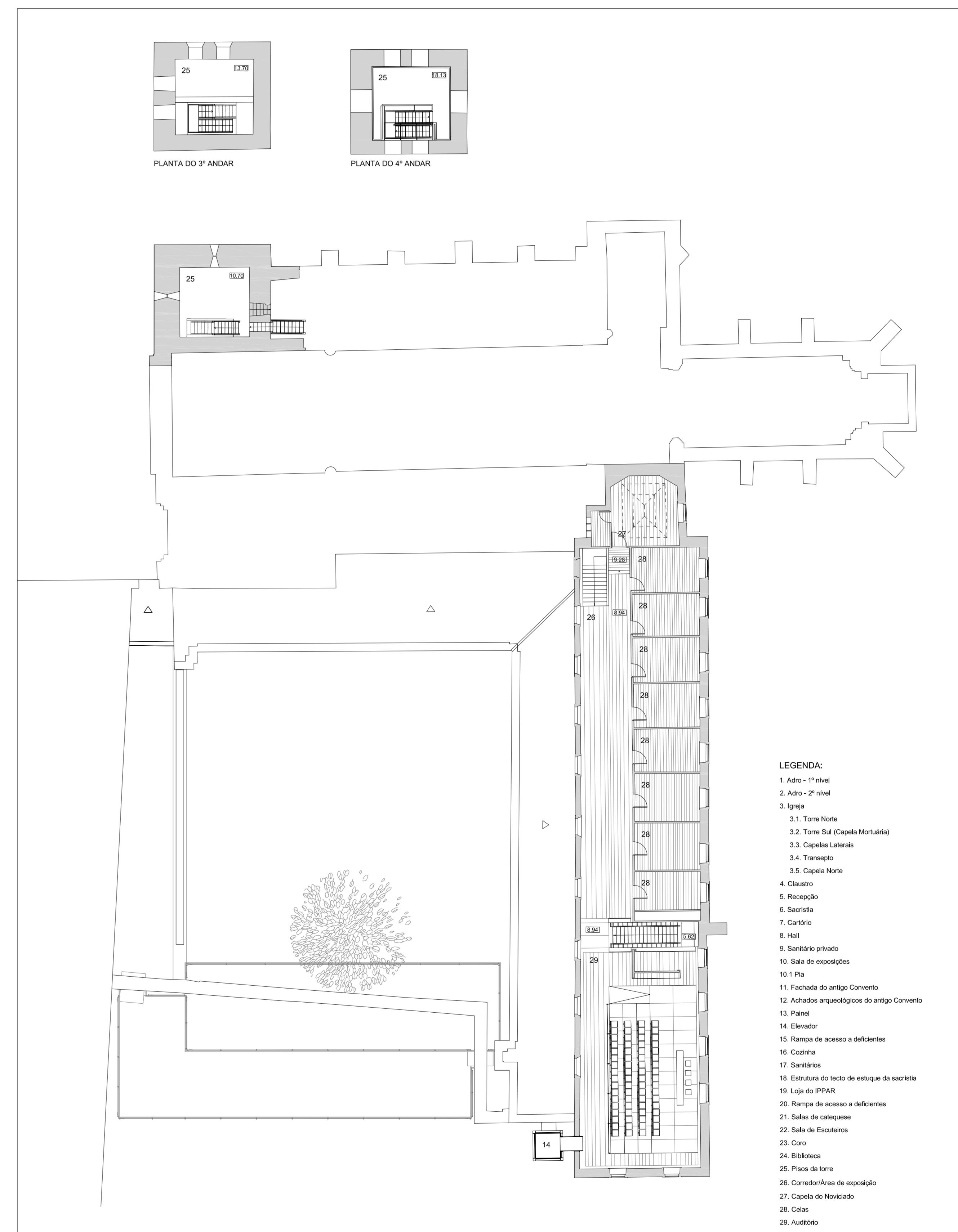
PLANTA DO 2º ANDAR PROPOSTA
