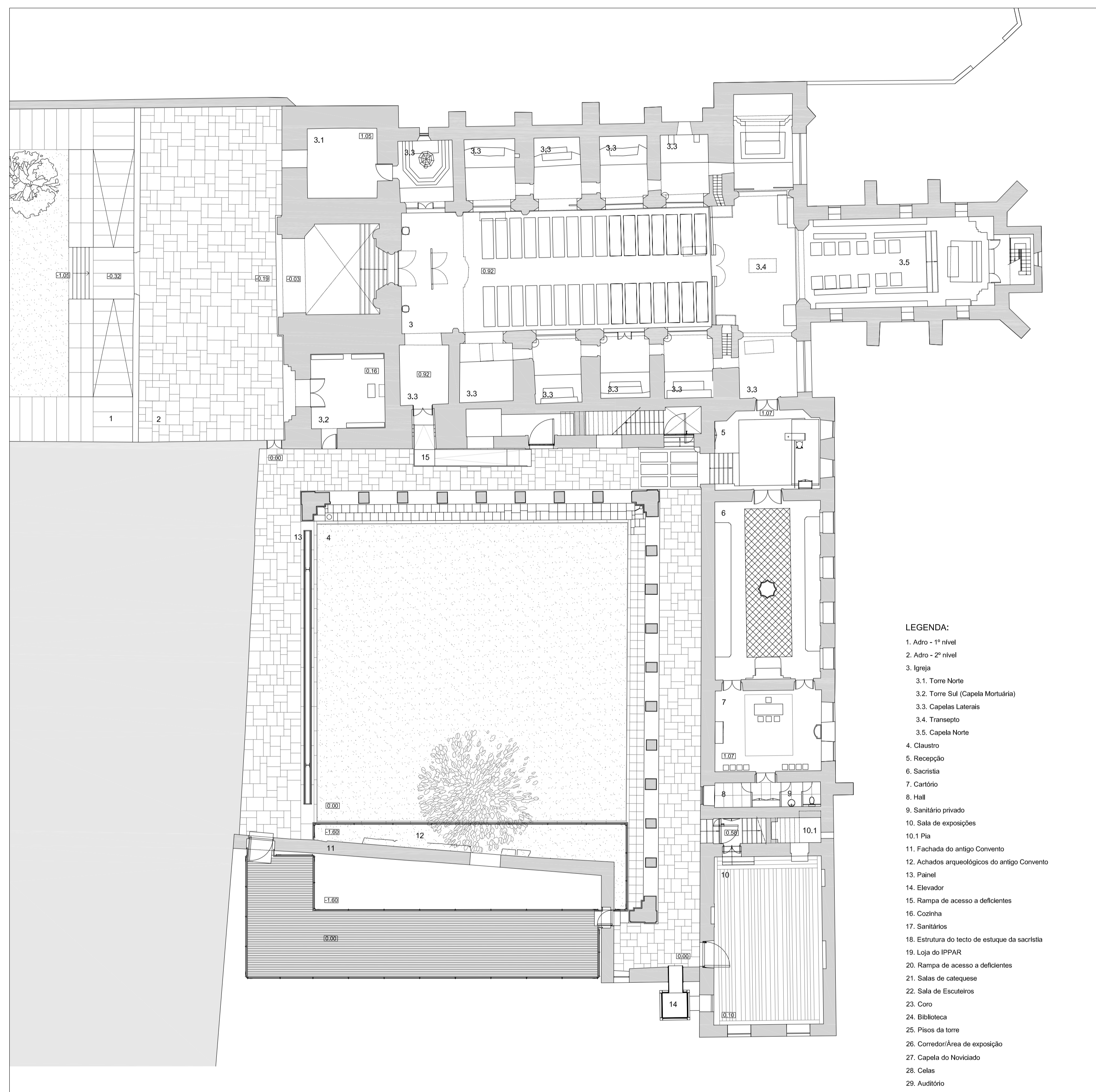
PLANTA DO PISO TÉRREO PROPOSTA
