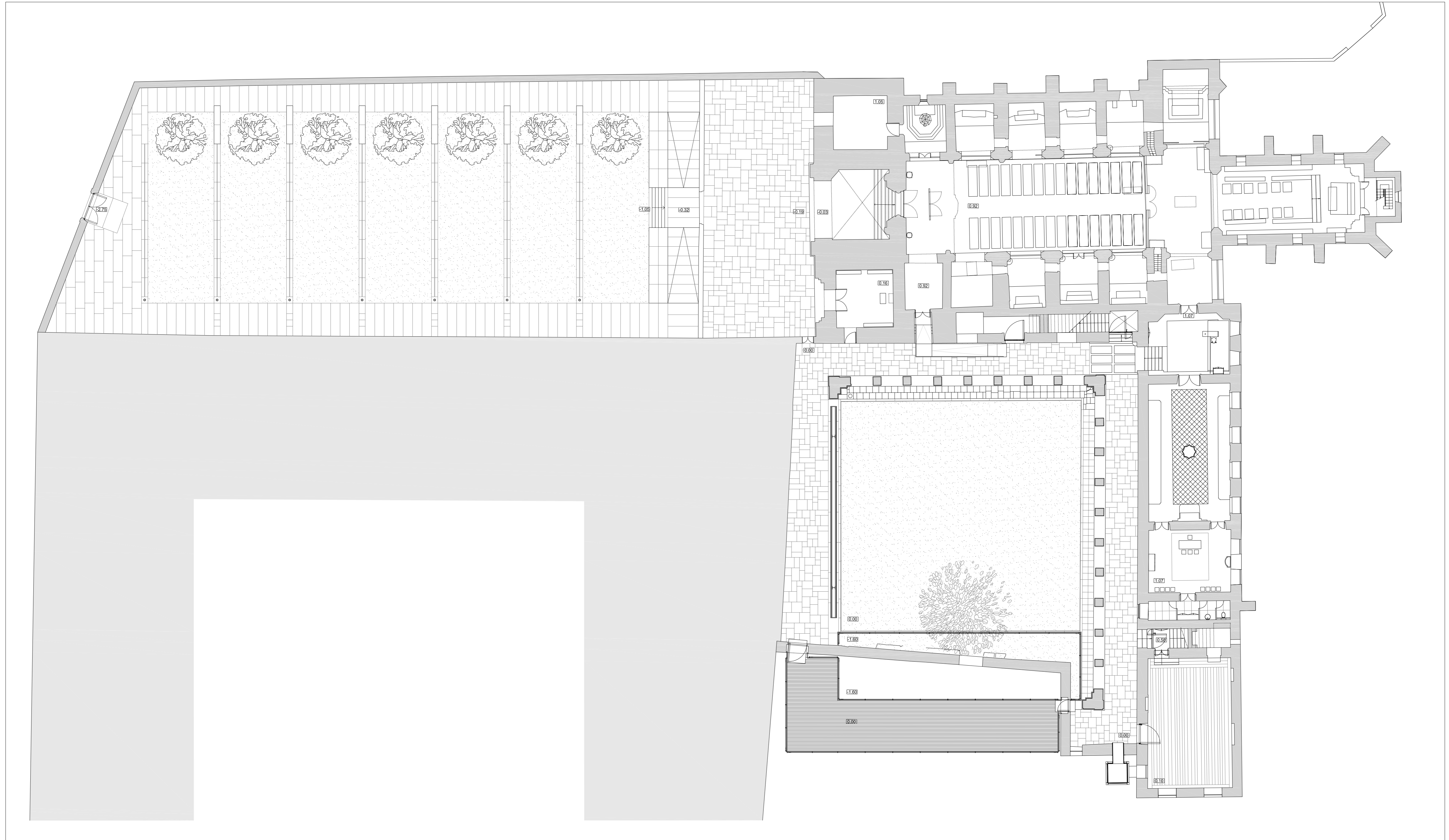
PLANTA GERAL DO PISO TÉRREO (PROPOSTA)
