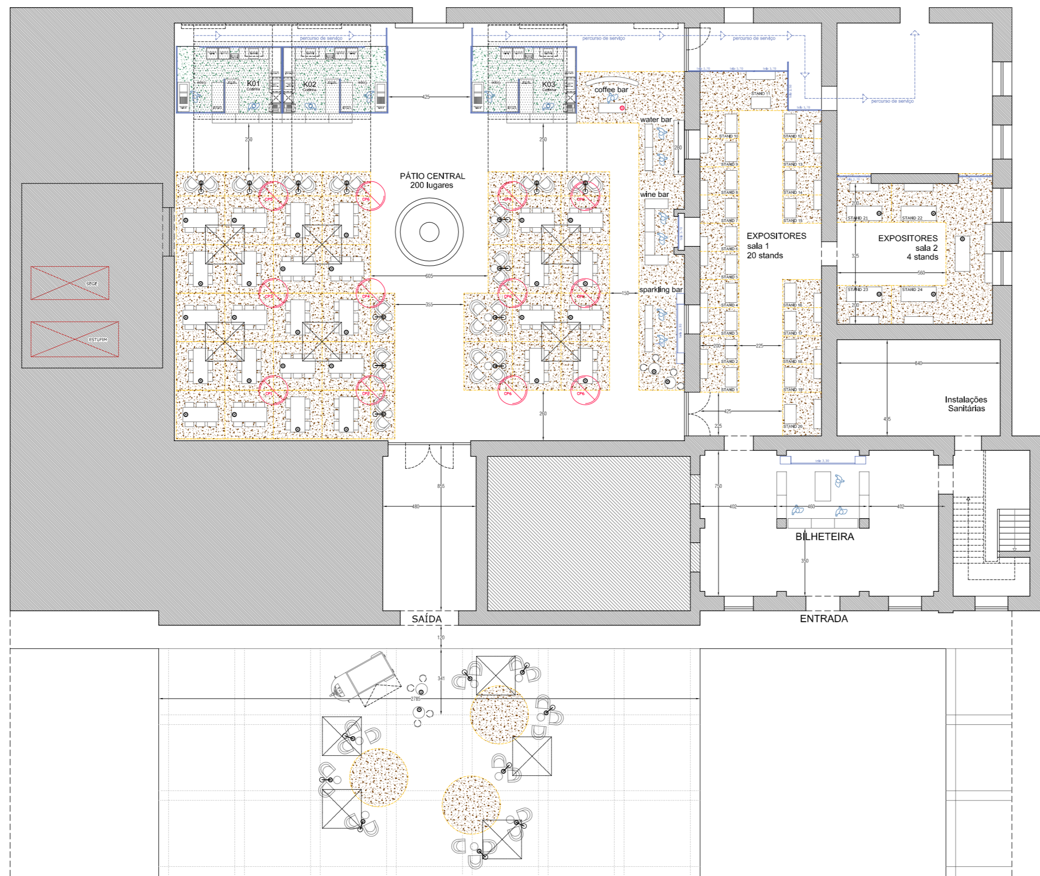
Planta de Rés-do-Chão
