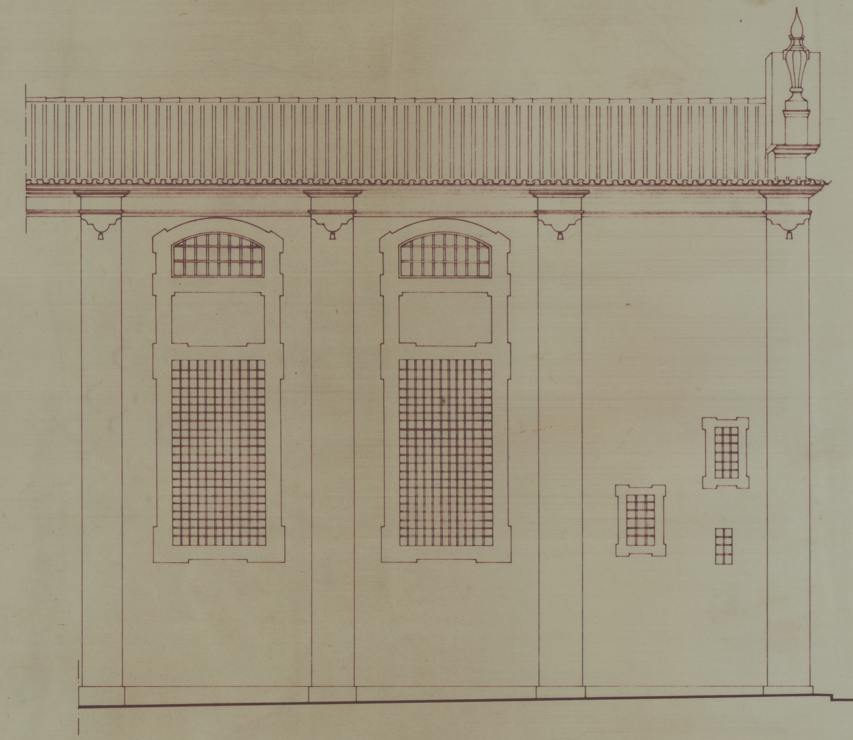
alçado sul
