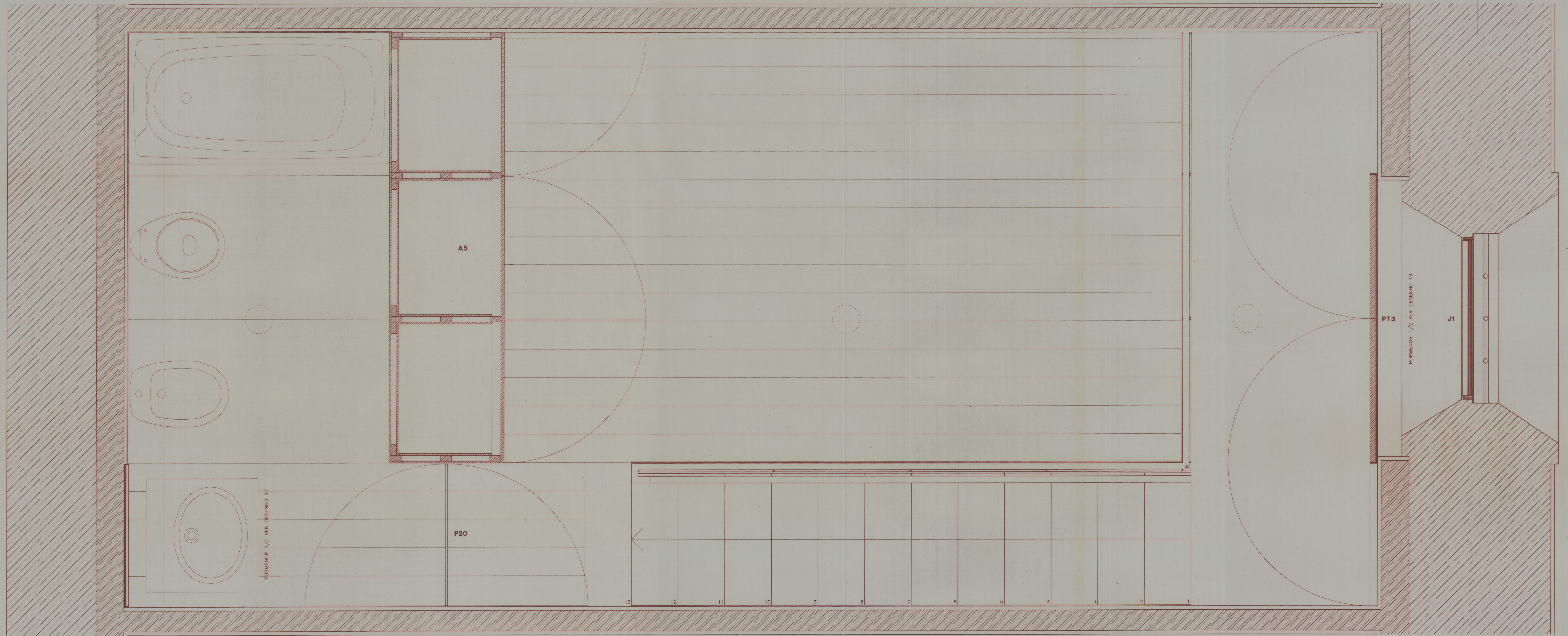
PLANTA DO QUARTO - ZONA DE DORMIR
