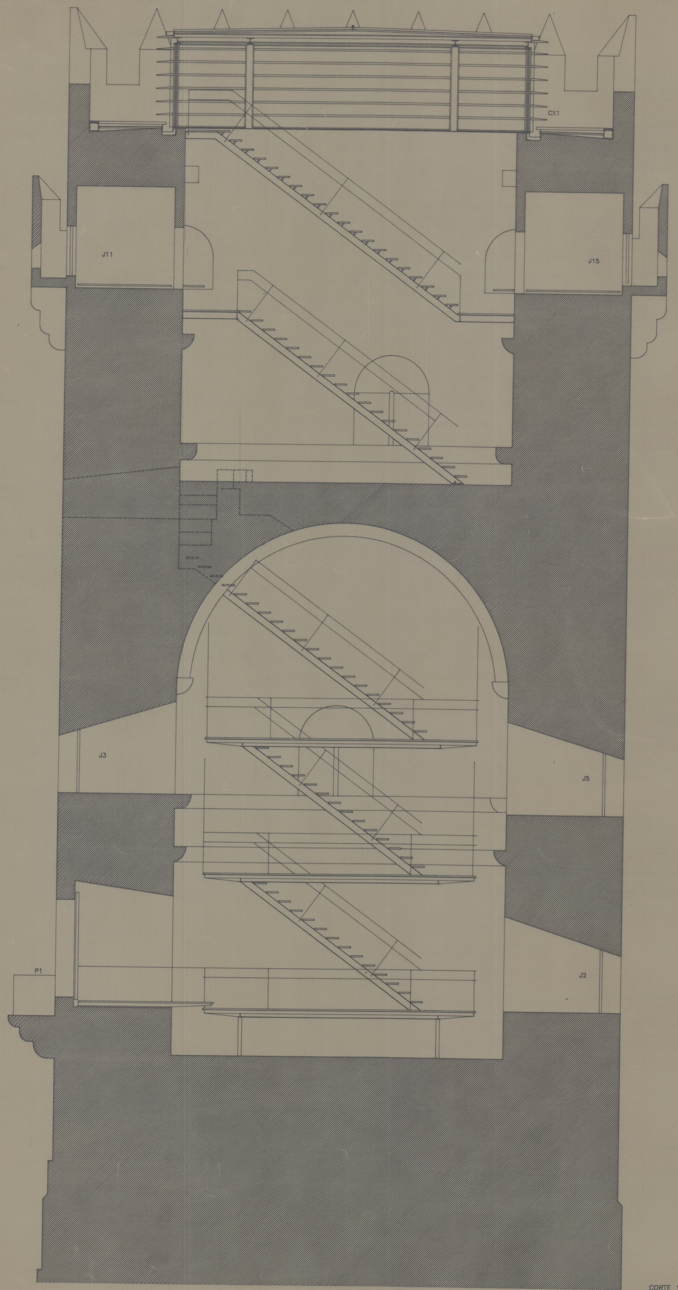
CORTE 1
