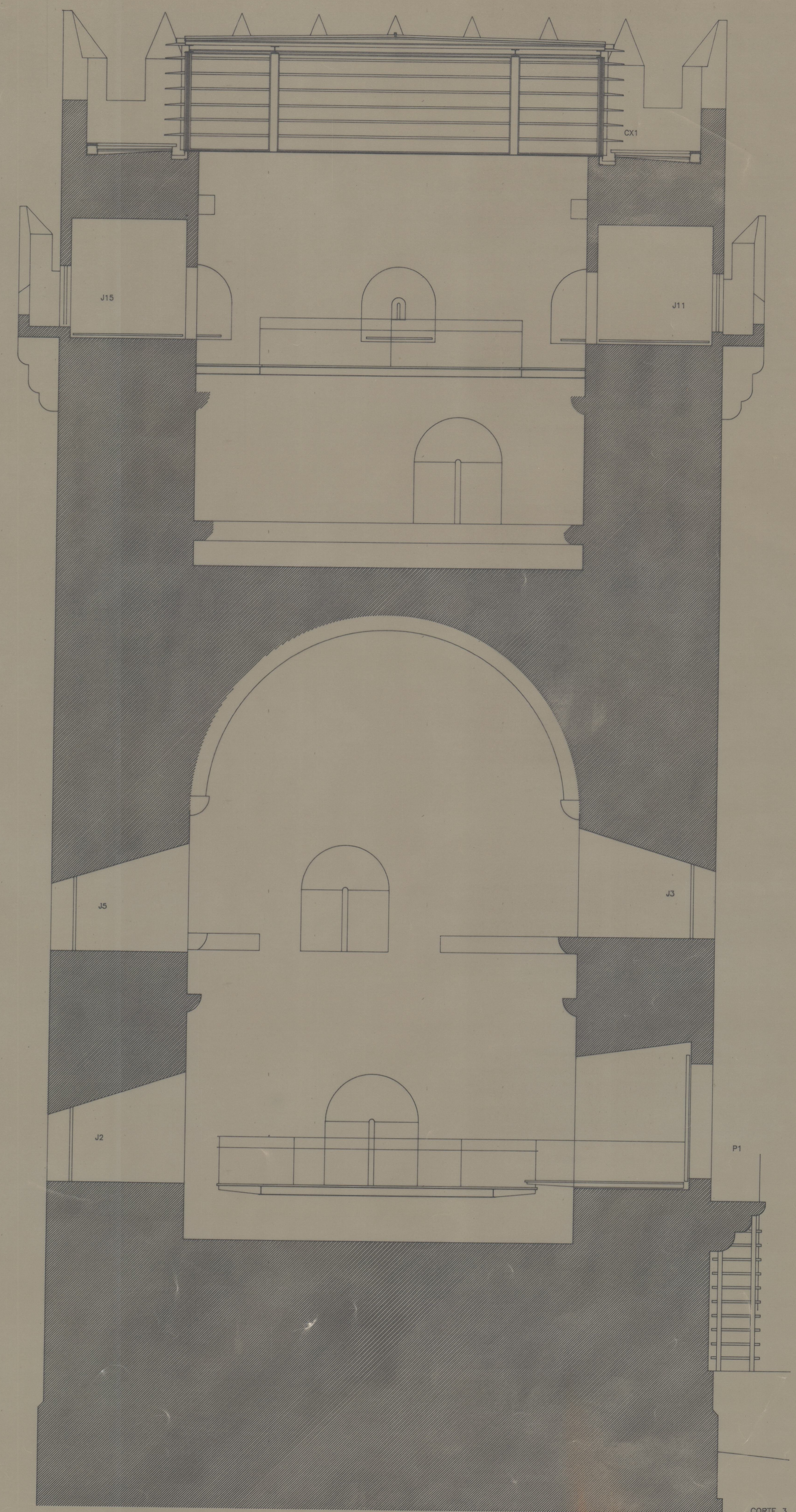
CORTE 3
