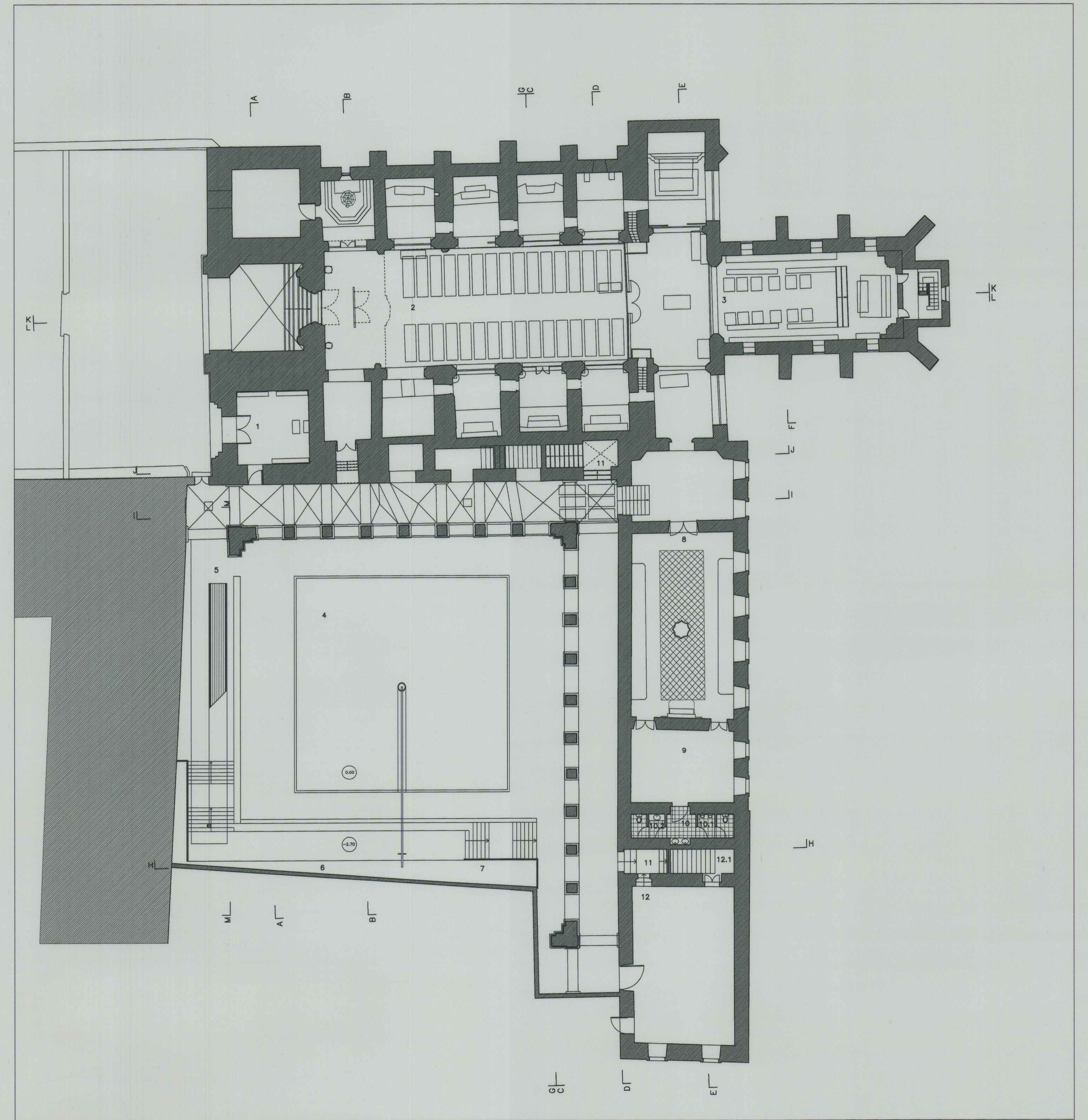
PLANTA DO PISO 0 . PROPOSTO
