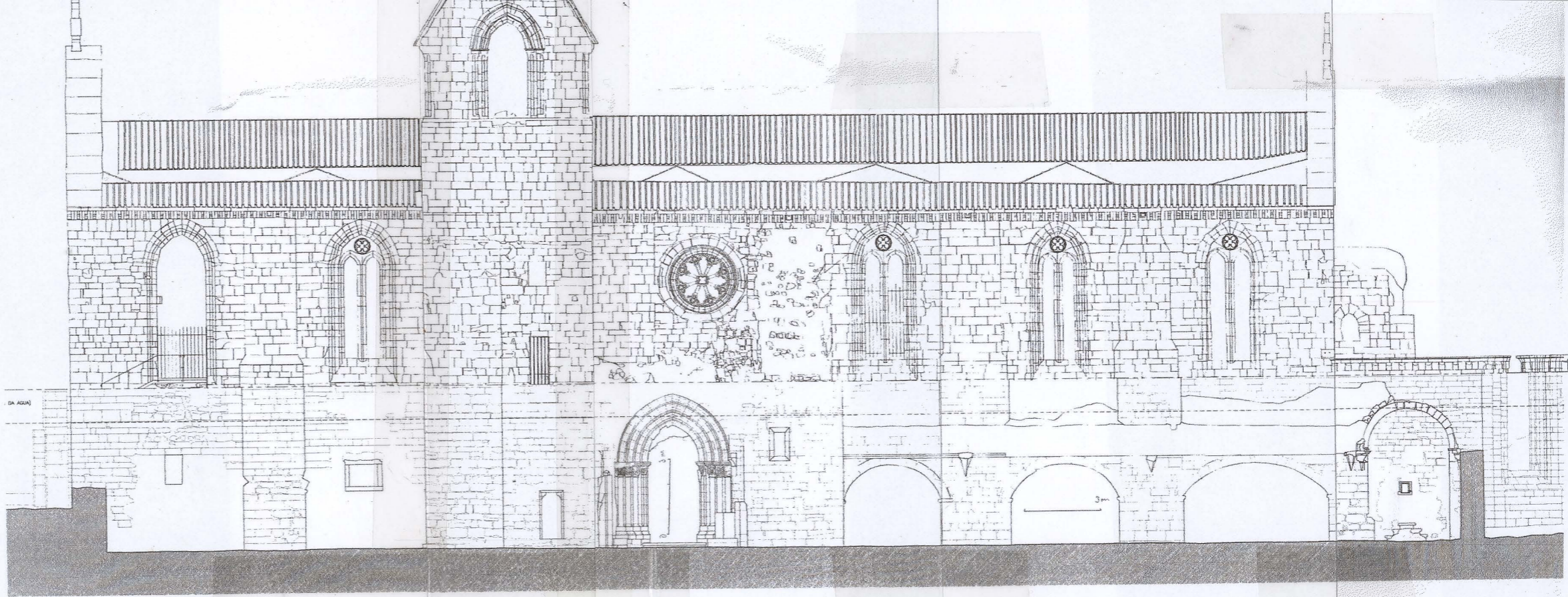
ALÇADO SUL
