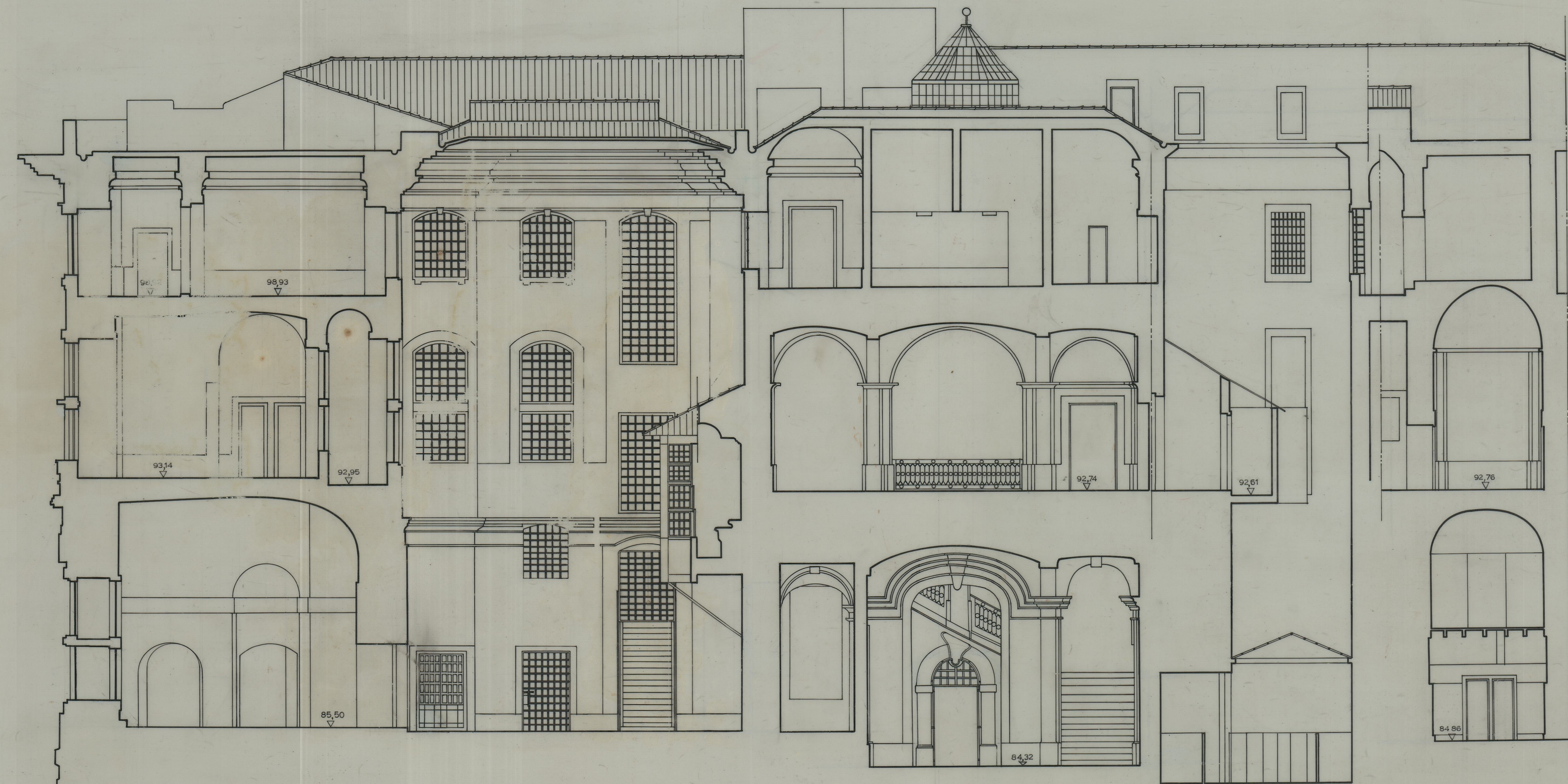
CORTE D-D'
