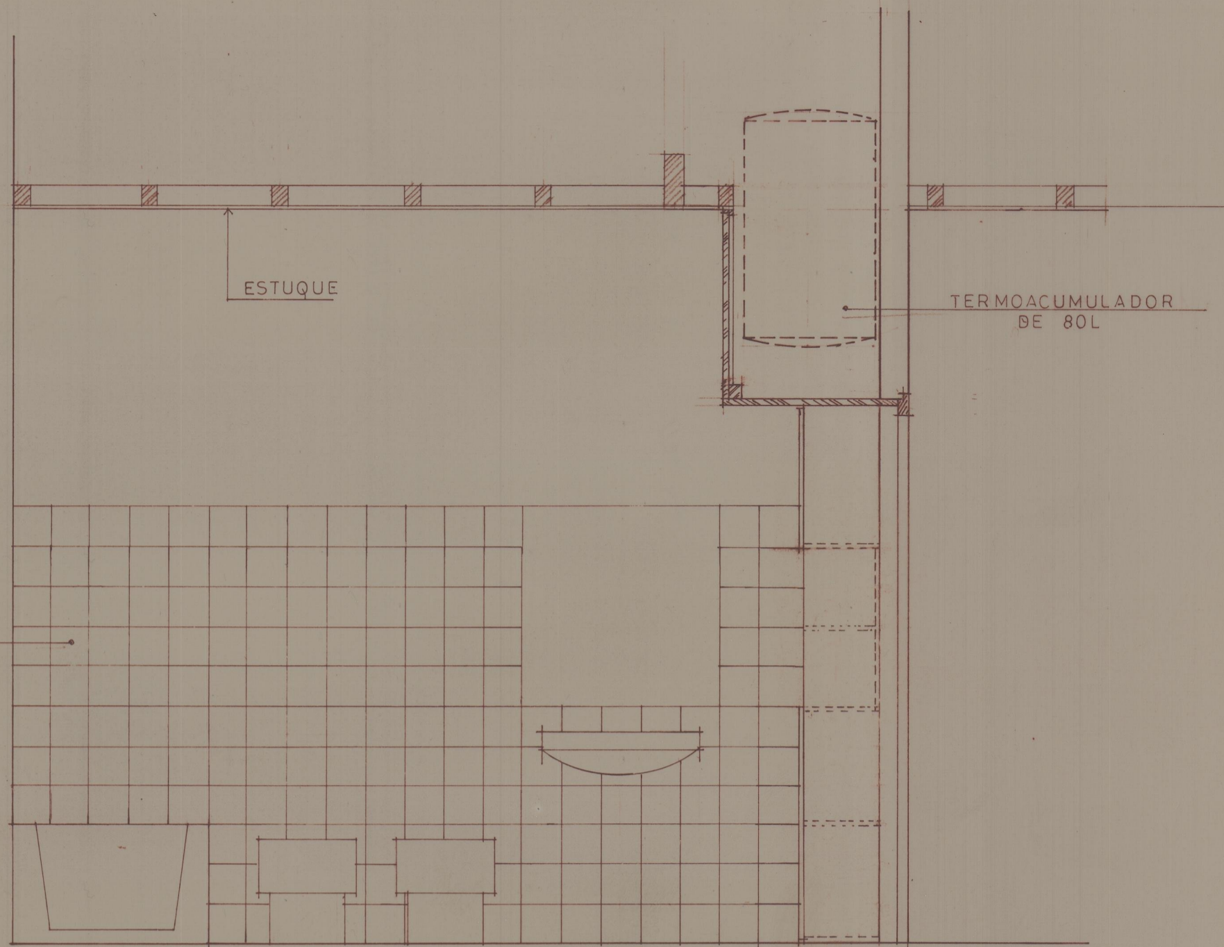
ALÇADO
