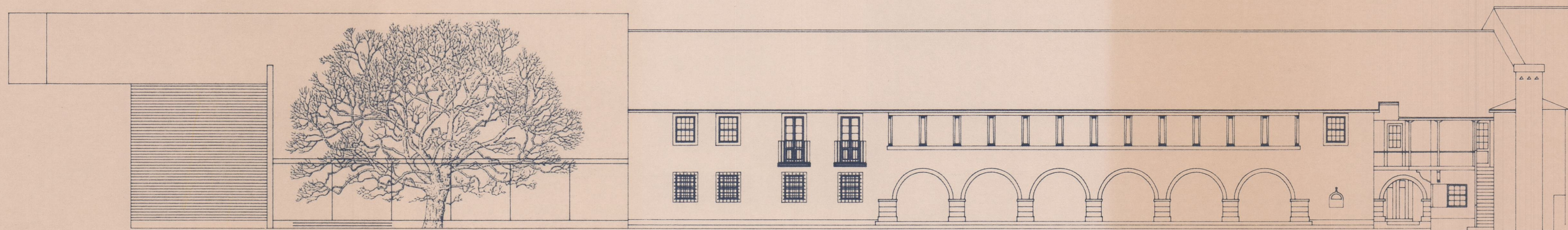
ALÇADO NORTE
