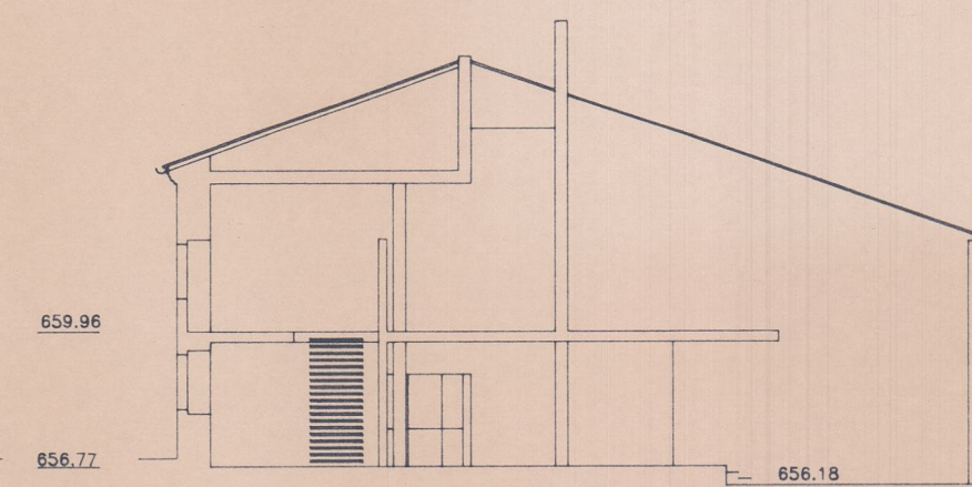
CORTE 4
