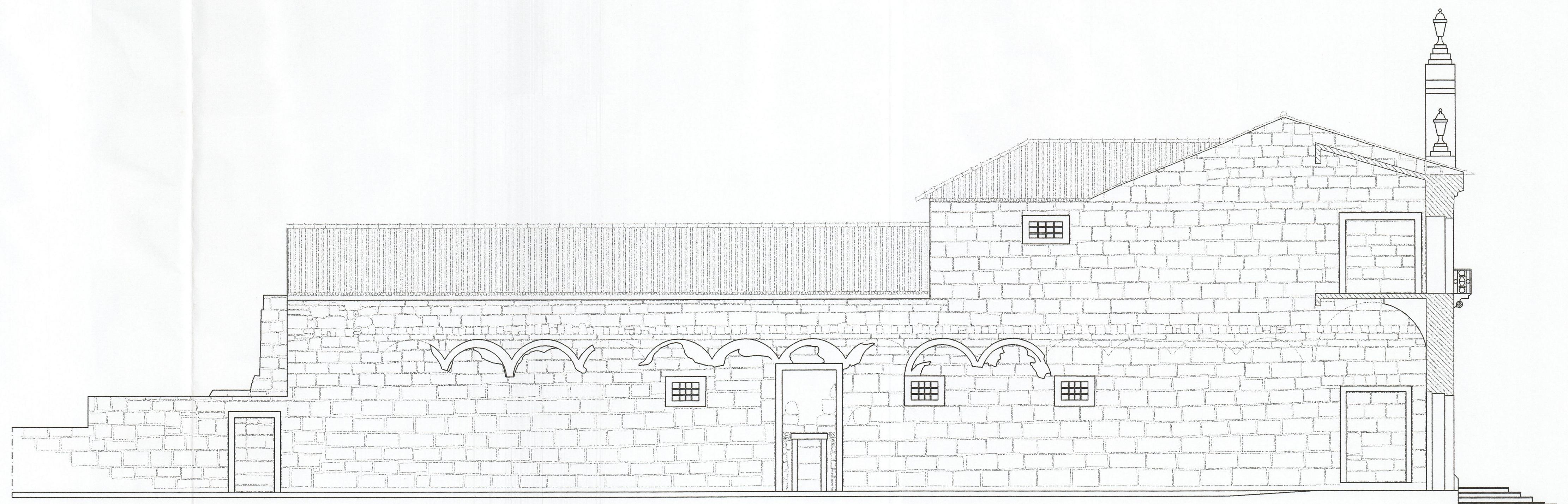
ALÇADO NASCENTE
