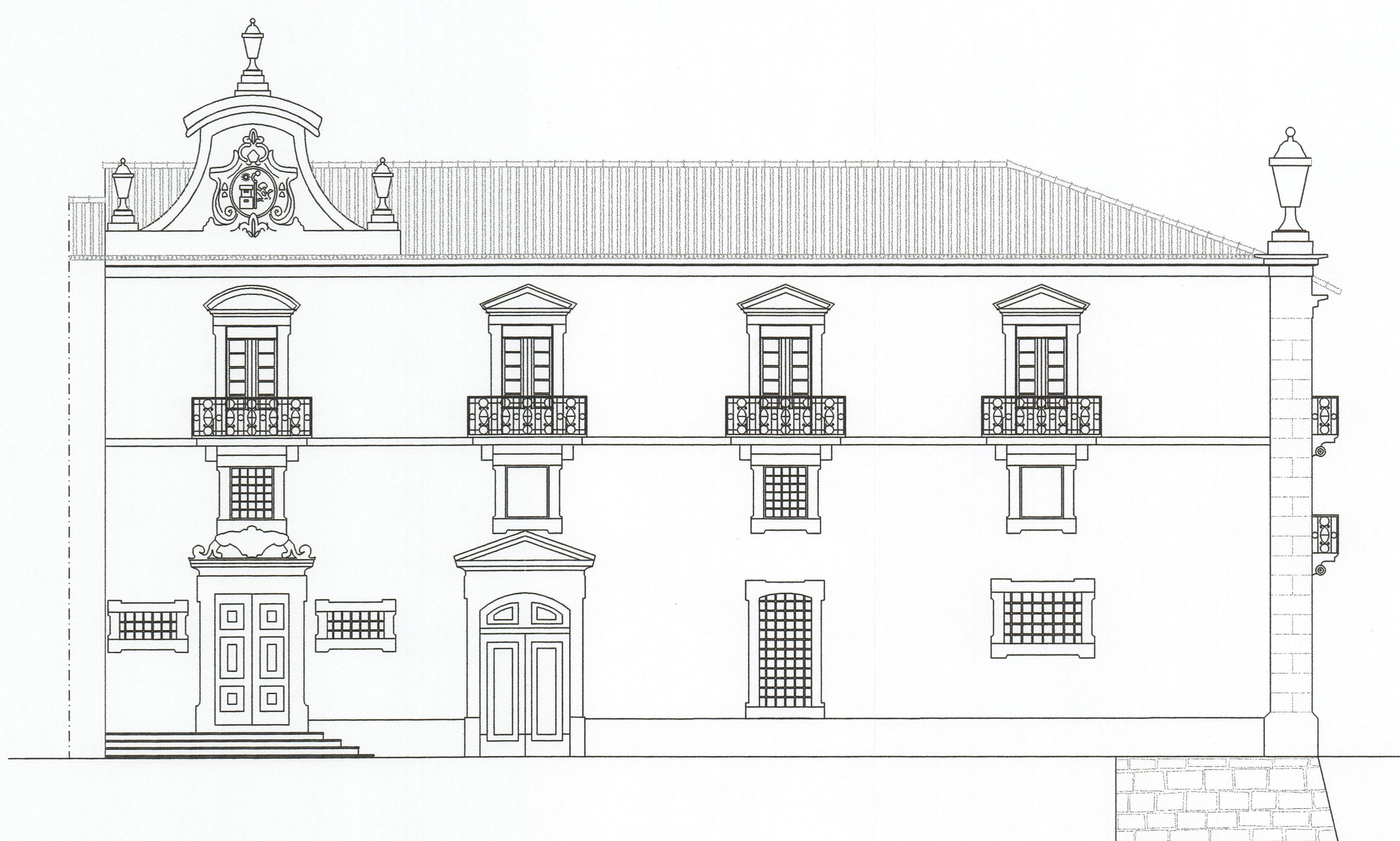
ALÇADO NORTE
