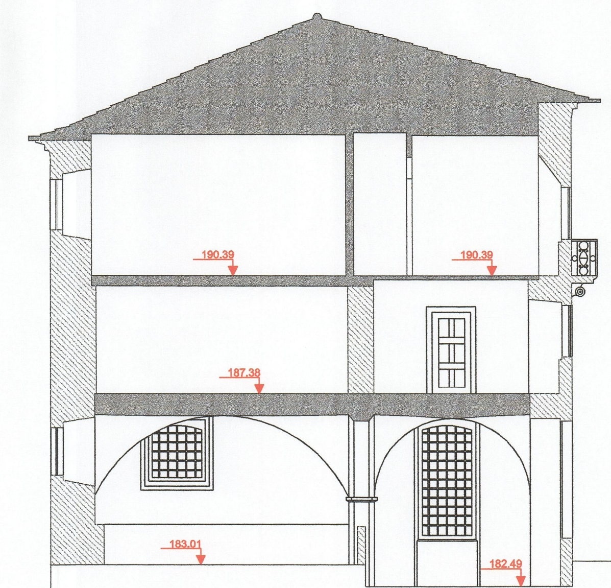
CORTE C' - D''
