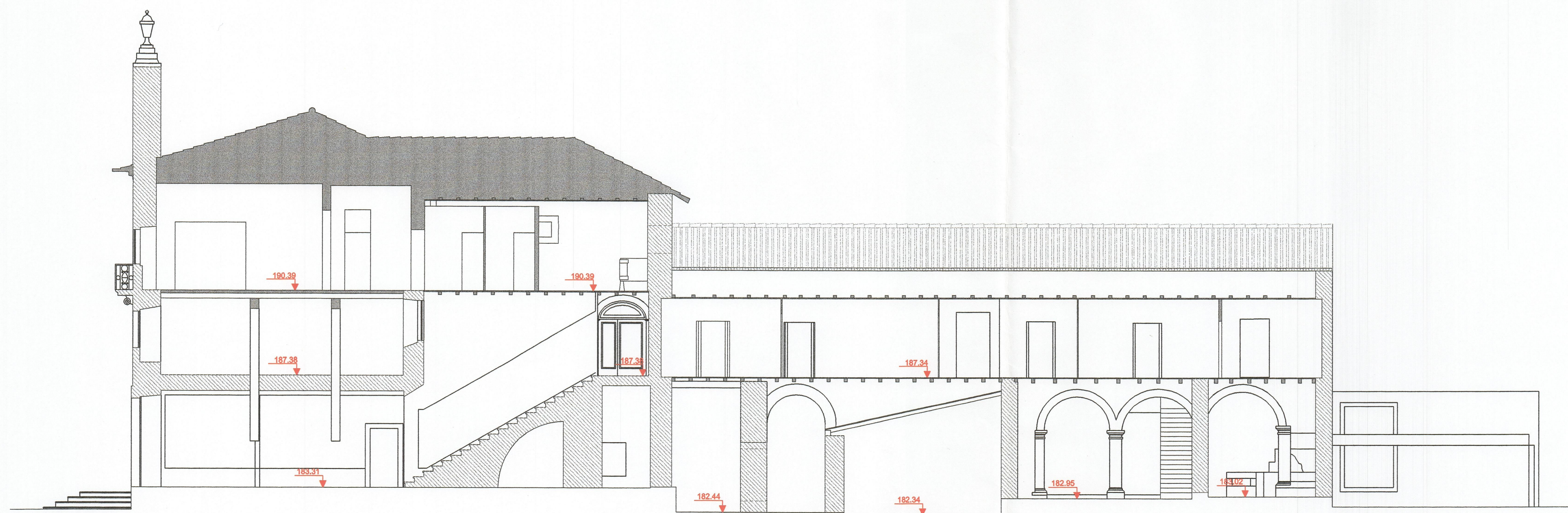
CORTE E - F
