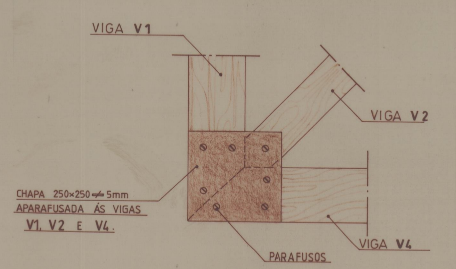
LIGAÇÃO DAS VIGAS V1, V2, V4 SOBRE OS PILARES (esc. 1/10)
