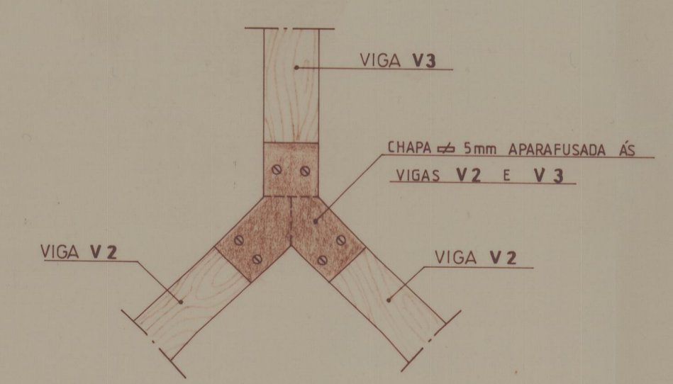
LIGAÇÃO NO ENCONTRO DAS VIGAS V2, V3 (esc. 1/10)
