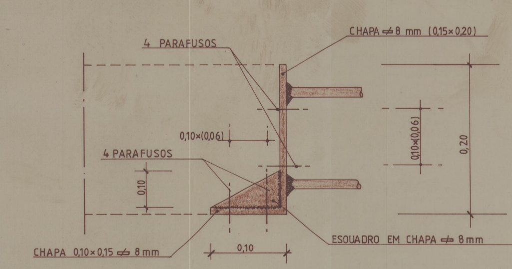
PORMENOR DO APOIO DAS VIGAS V1 (esc. 1/5)
