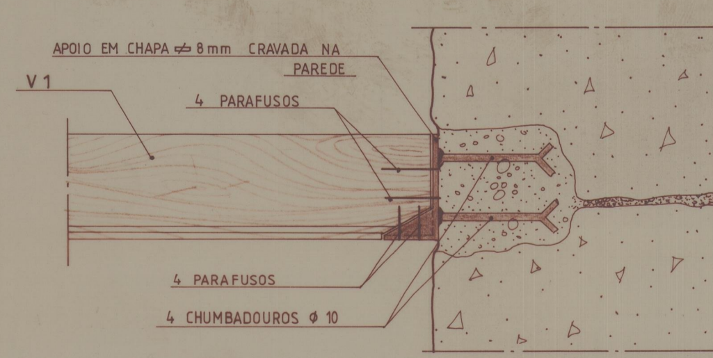
APOIO DAS VIGAS V1 NA PAREDE (esc. 1/10)
