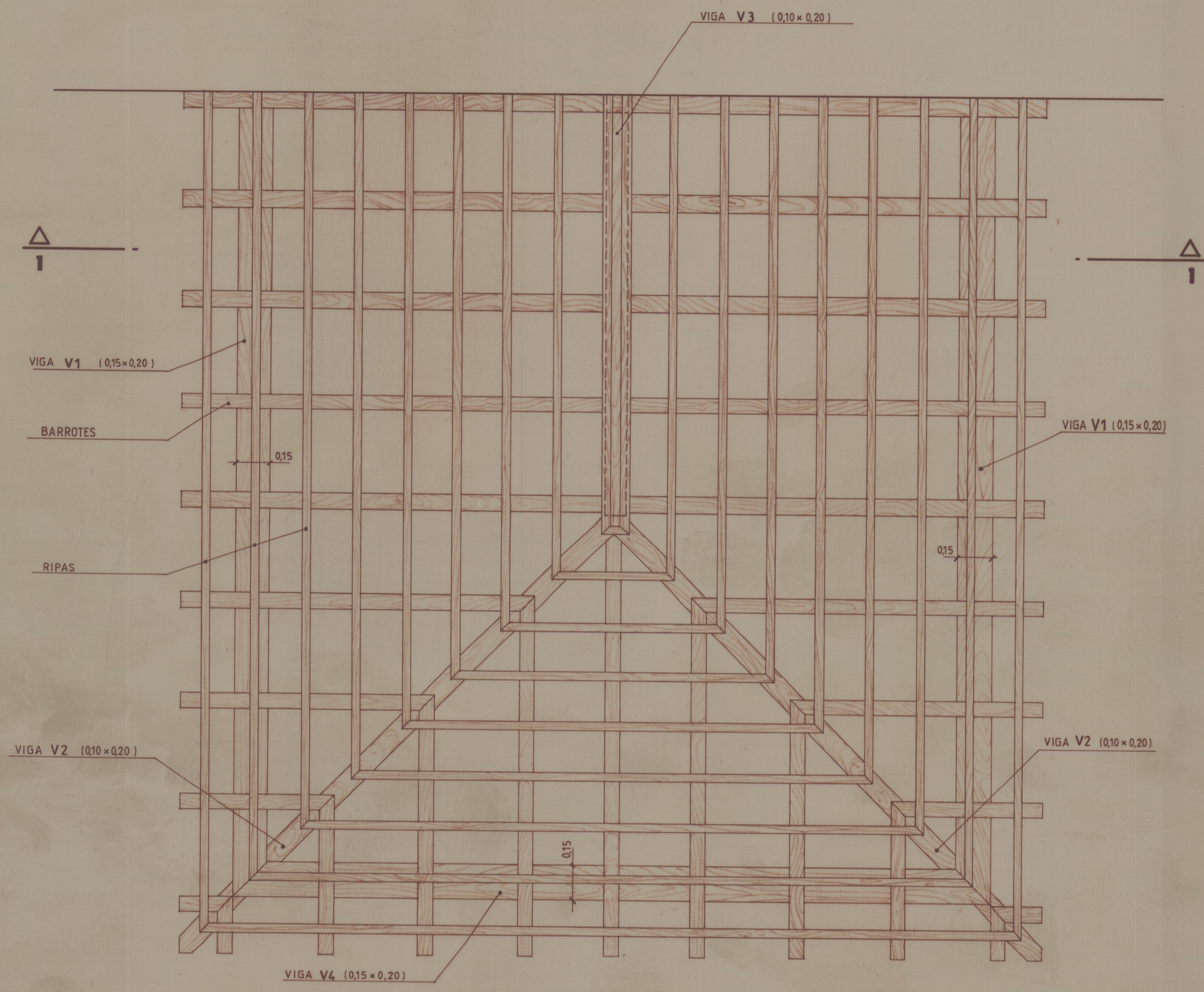
PLANTA ESQUEMÁTICA DA COBERTURA (esc. 1/20)
