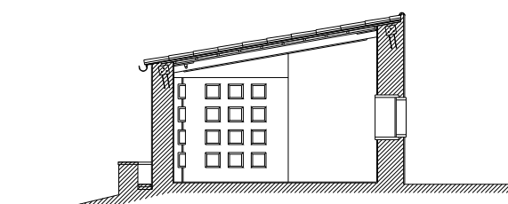
CORTE 3-4
