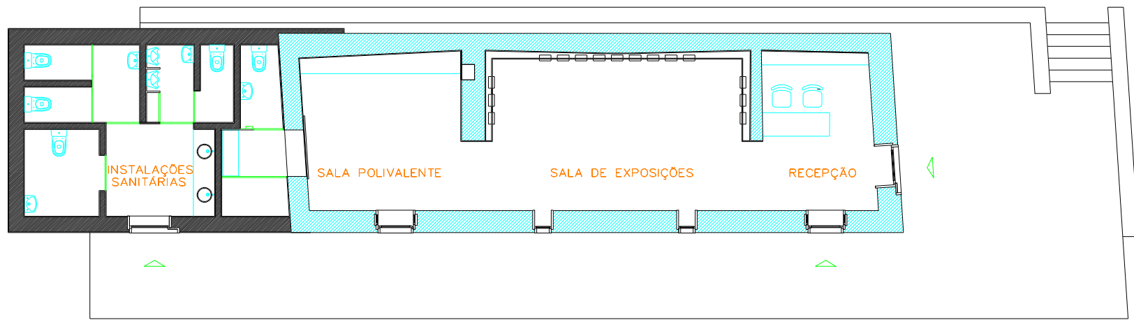
PLANTA
