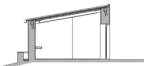
CORTE 1-2
