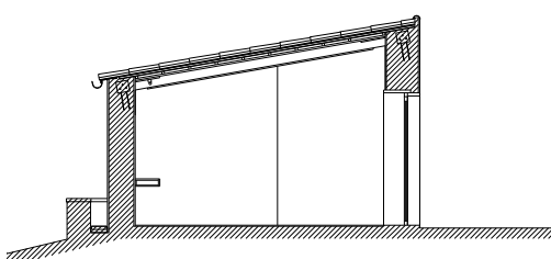
CORTE 1-2
