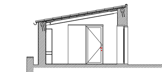
CORTE 5-6
