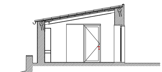
CORTE 5-6
