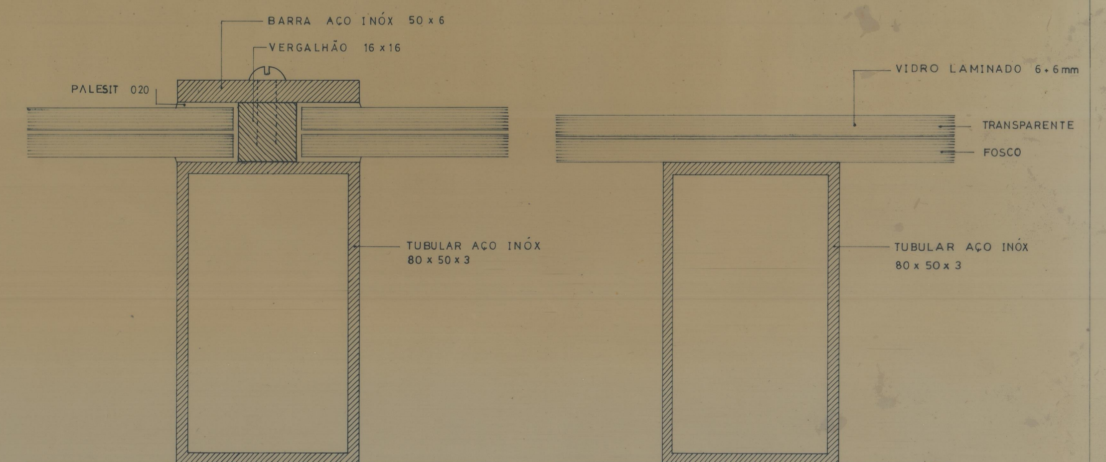
PORM 5 ESC. 1:1
