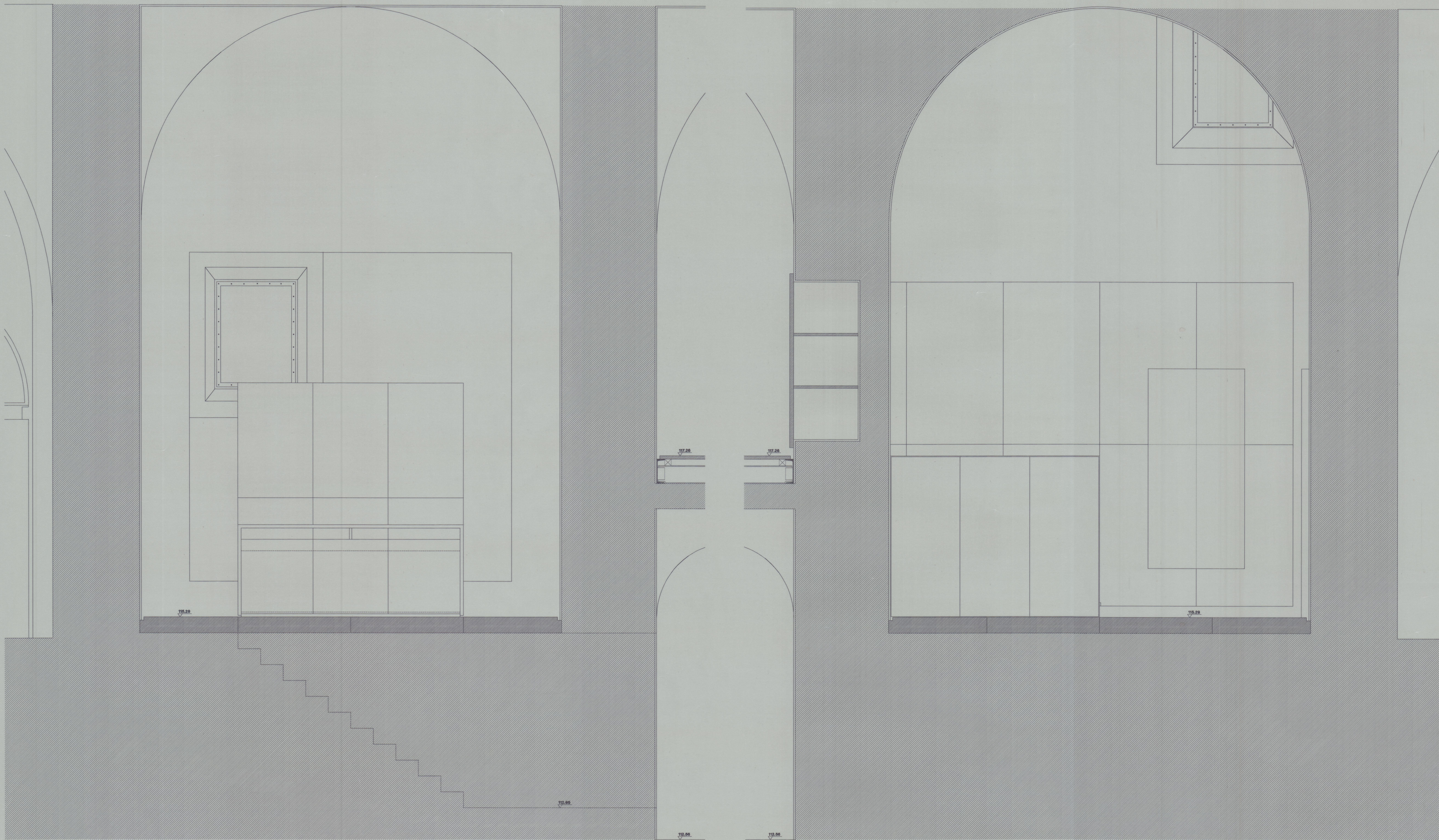
Corte 5
