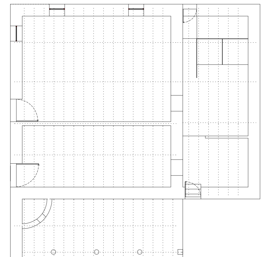
PLANTA DE DISTRIBUIÇÃO (VIGAS E BARROTES)
