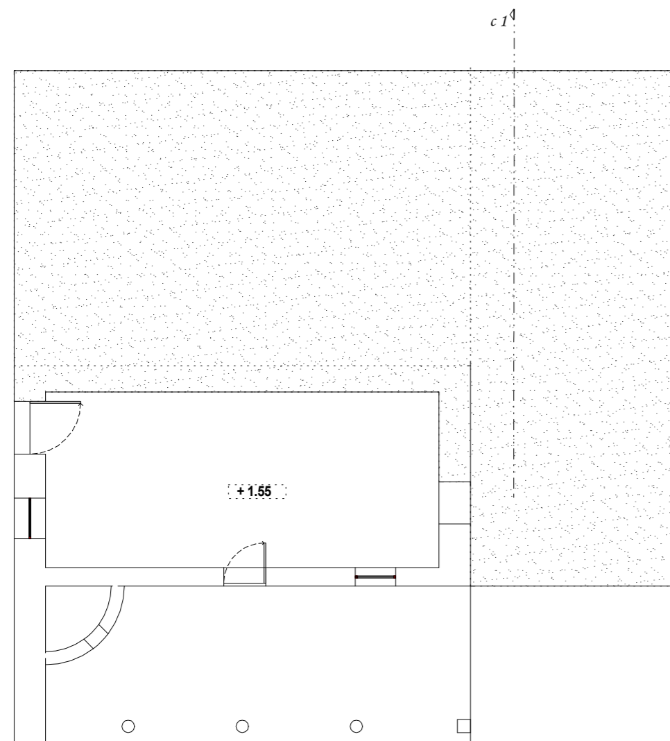
PLANTA DA CAVE
