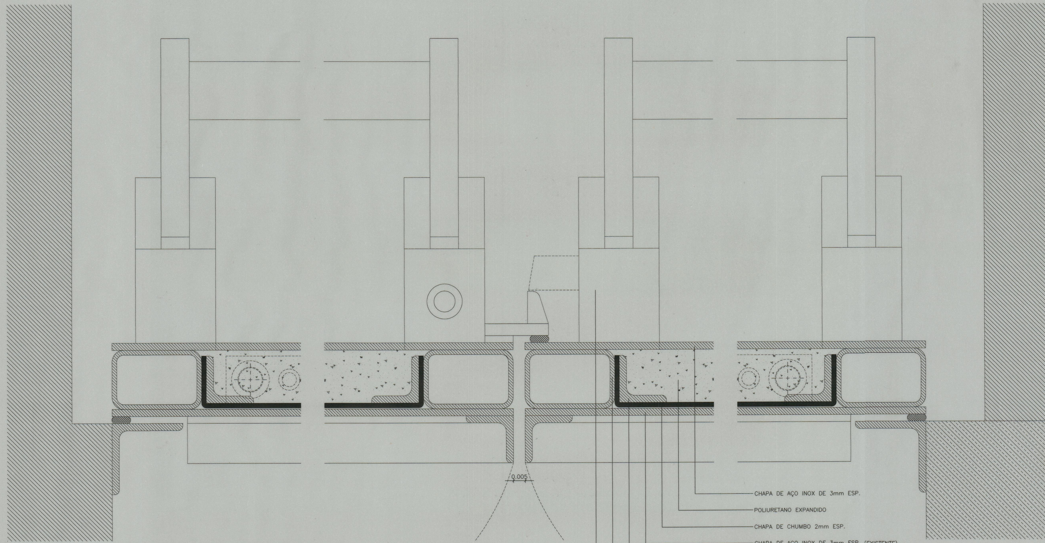
CORTE HORIZONTAL
