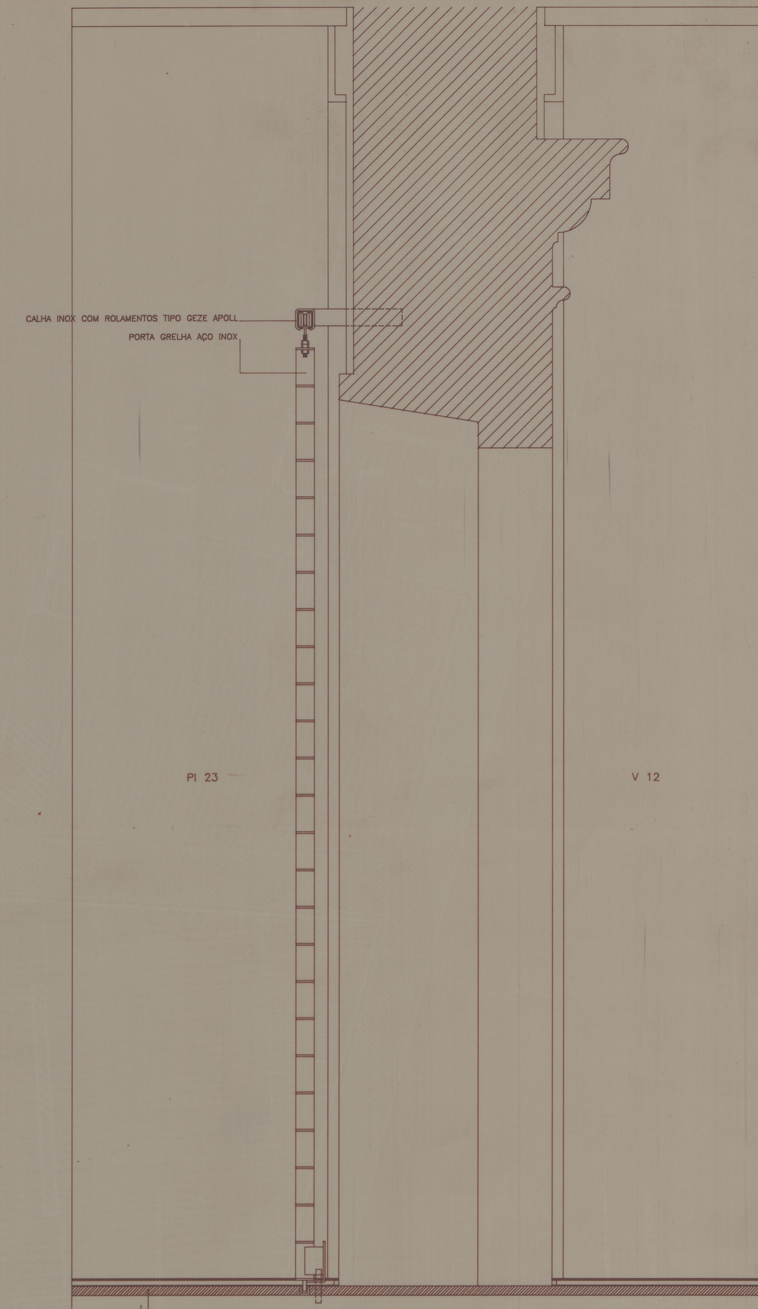
CORTE 3
