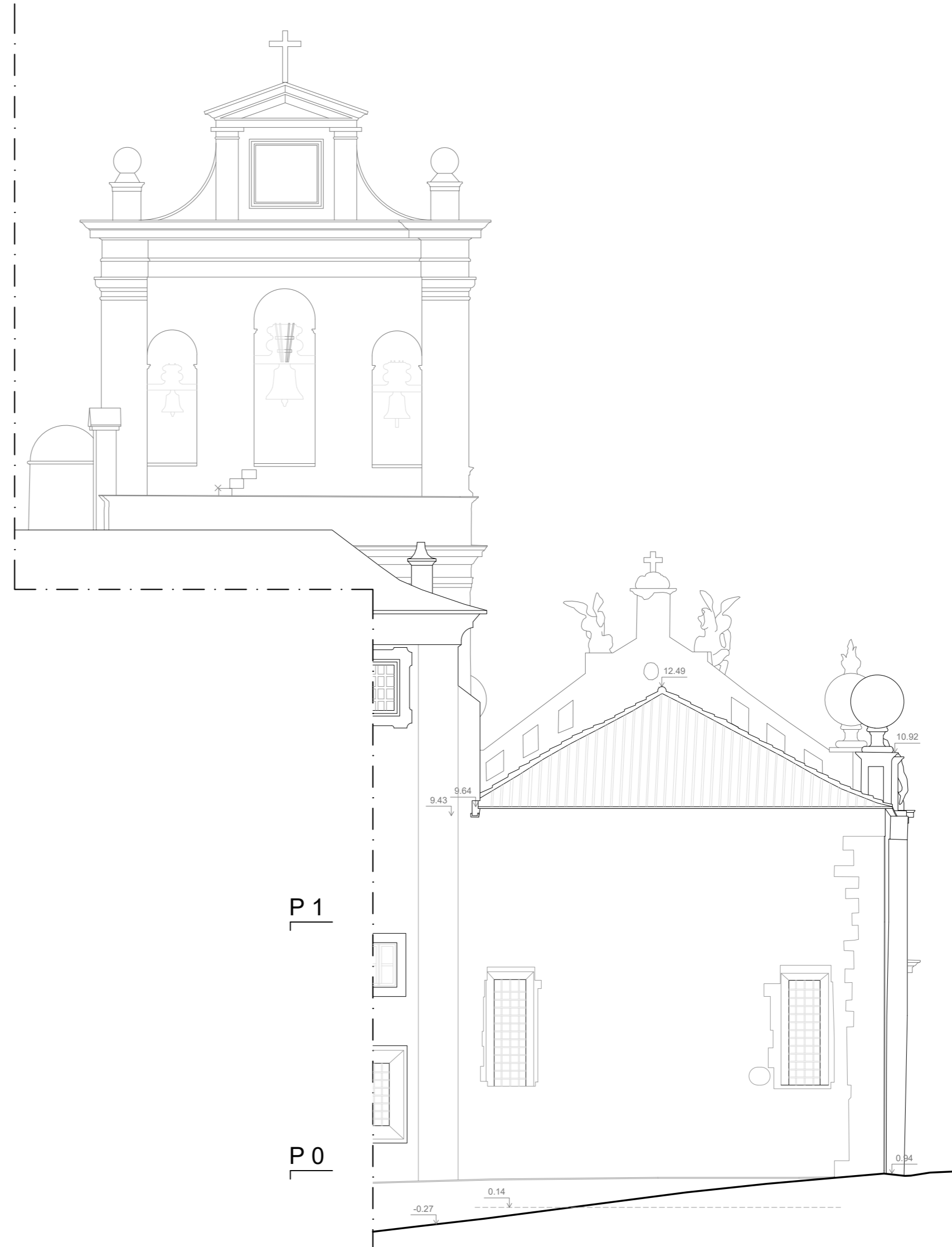
Alçado Posterior
