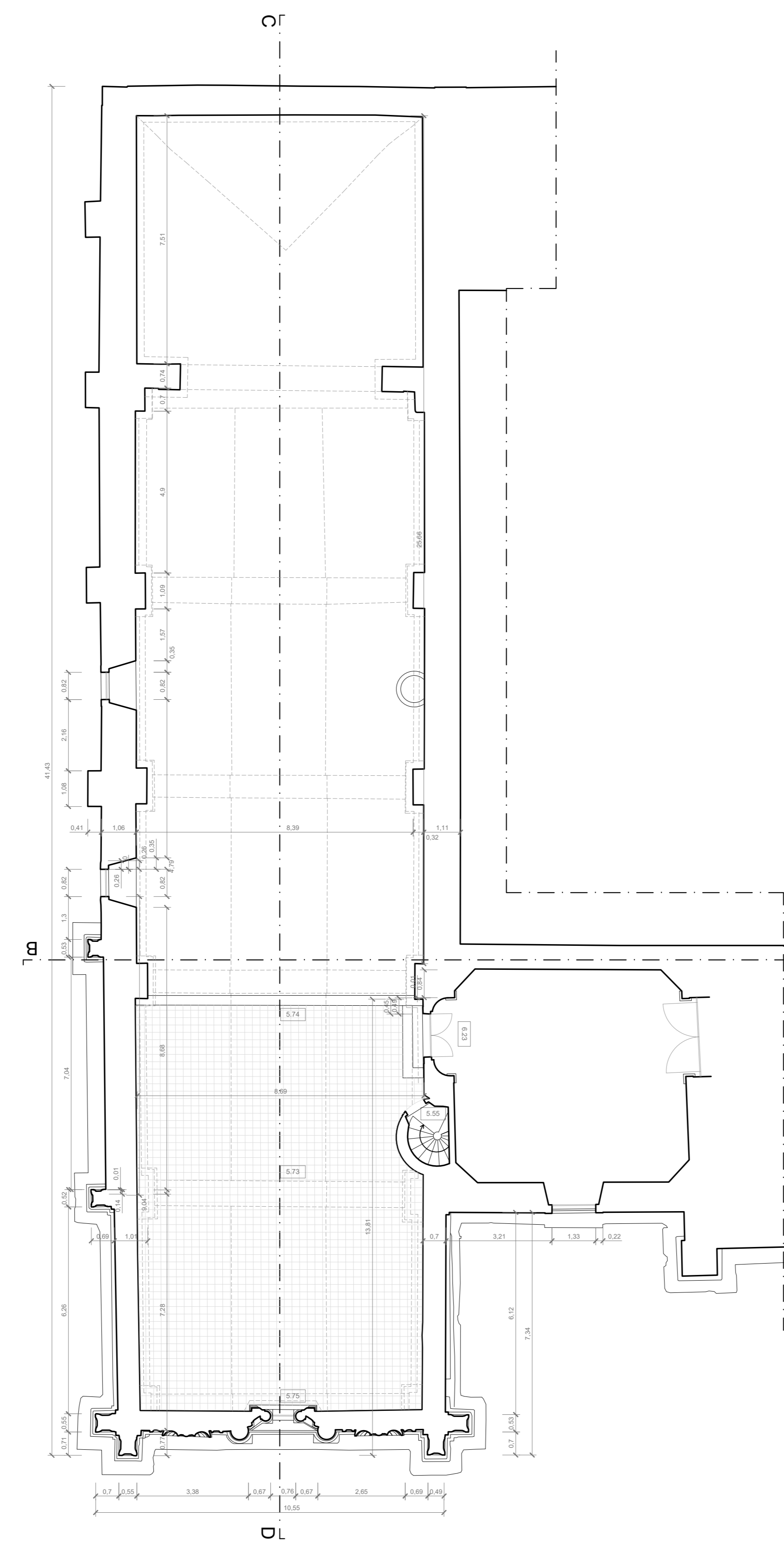
Planta Piso 1
