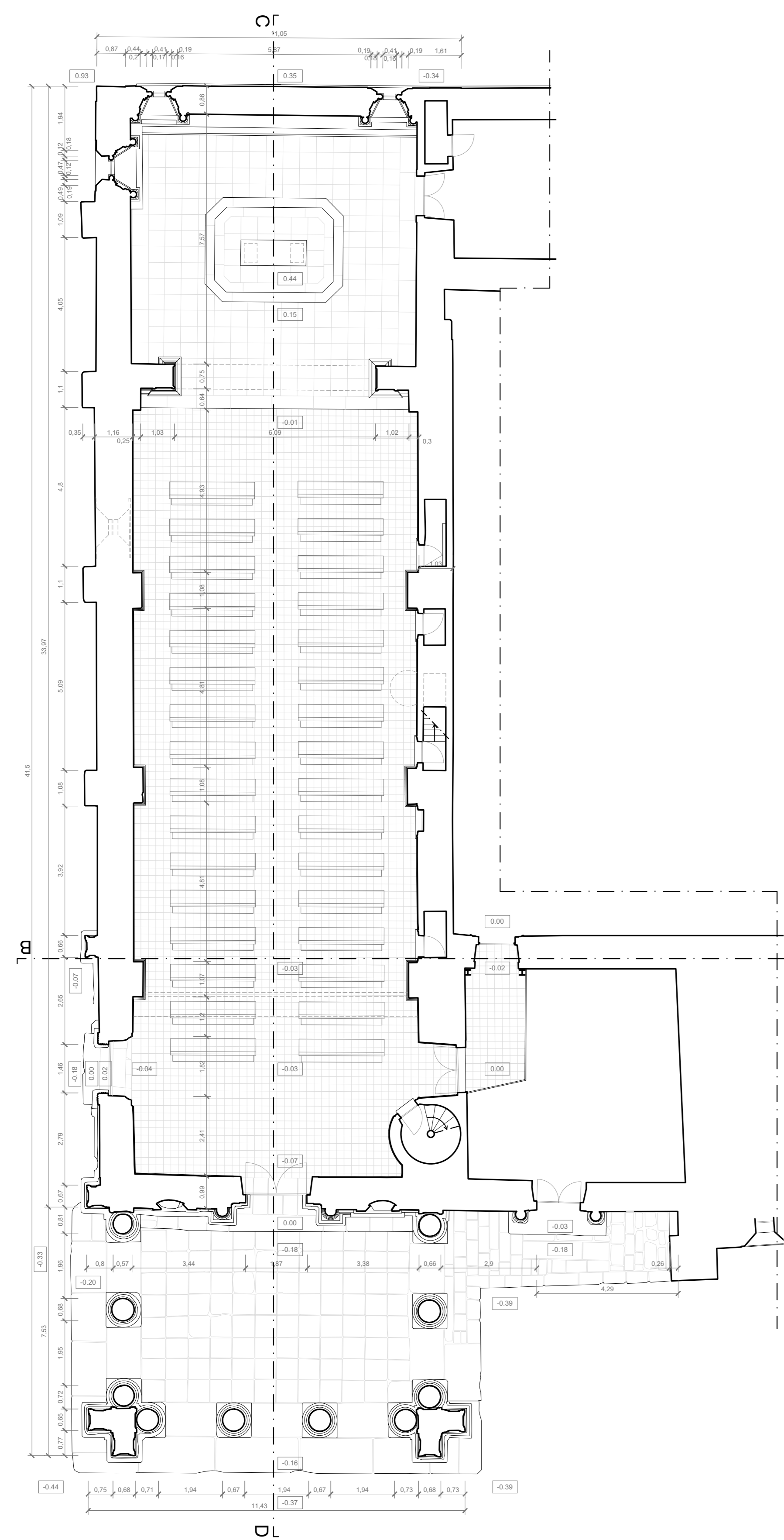
Planta Piso 0
