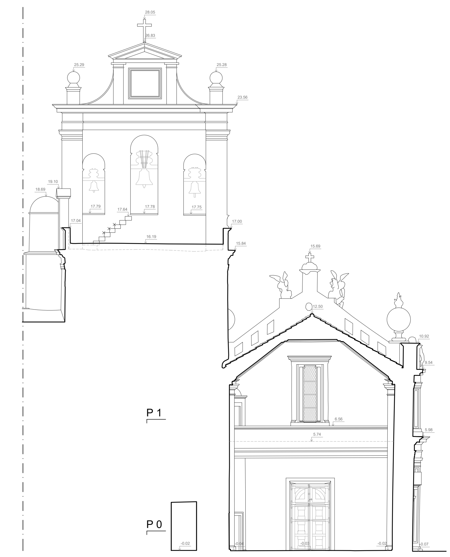
Corte A-B
