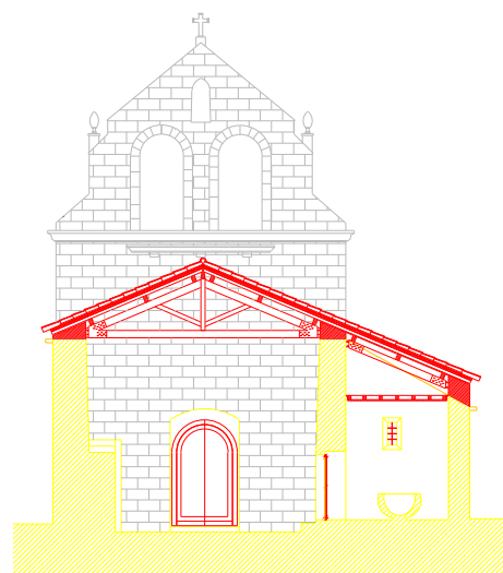
Corte 3 . 3
