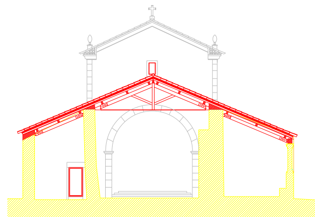
Corte 5 . 5
