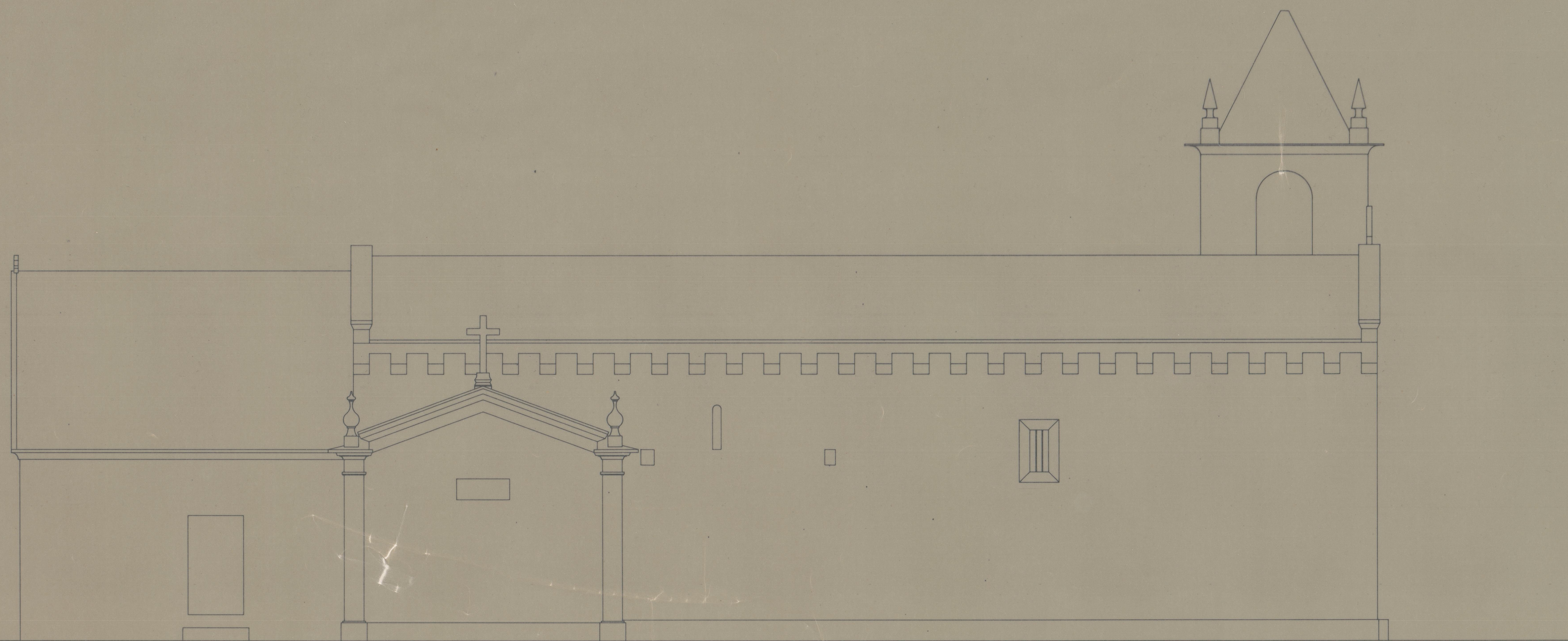
ALÇADO NORTE
